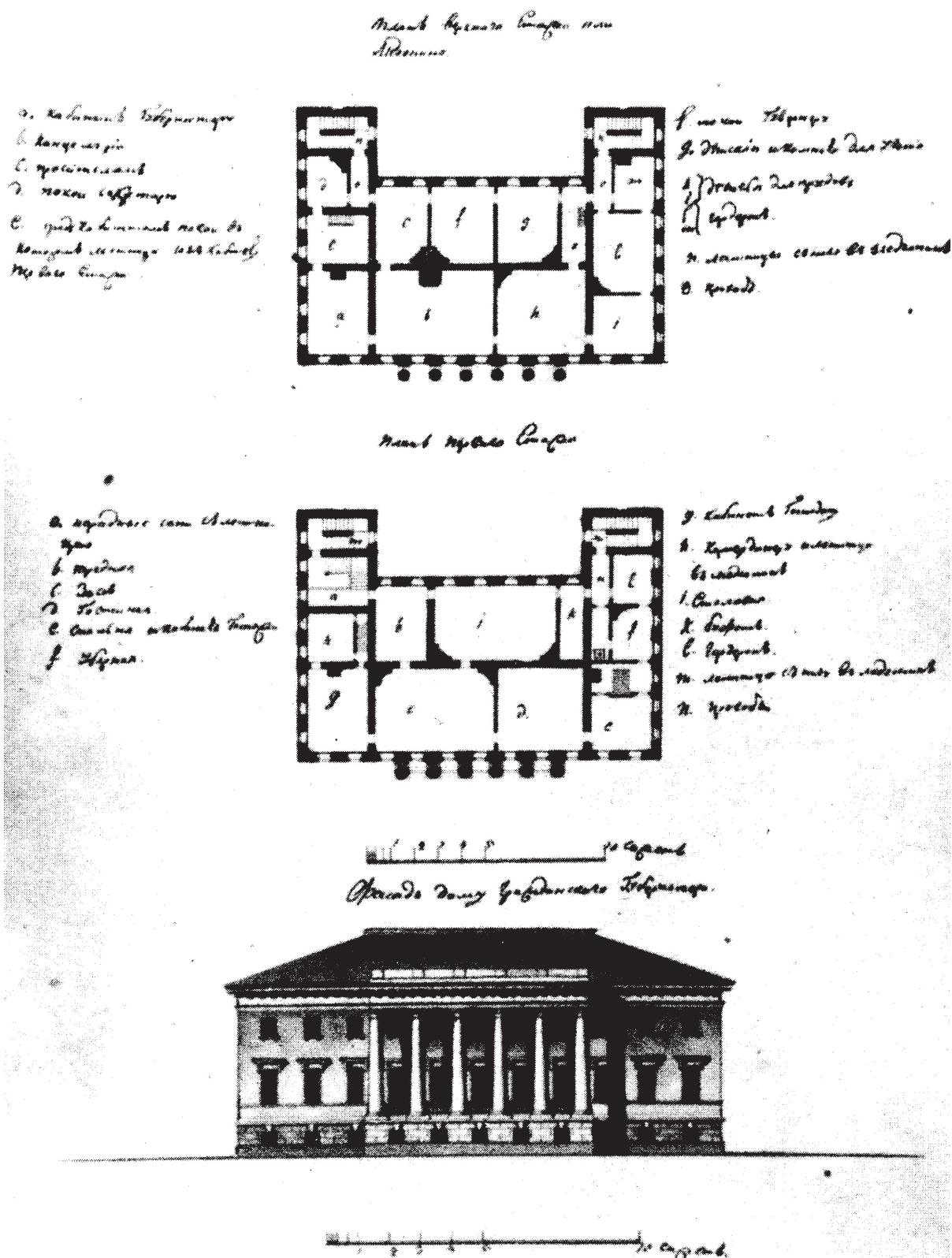
Рис. 1. Типовой проект дома гражданского губернатора для губернских городов. Архитектор А. Захаров. 1803 г. [126]
