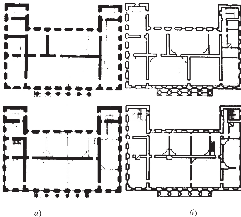
Рис. 2. Сопоставление планов 1-го и 2-го этажей дома гражданского губернатора типового проекта (а) и 2-го и 3-го этажей дома губернатора во Владимире (б). Реконструкция С.А. Муращенко
