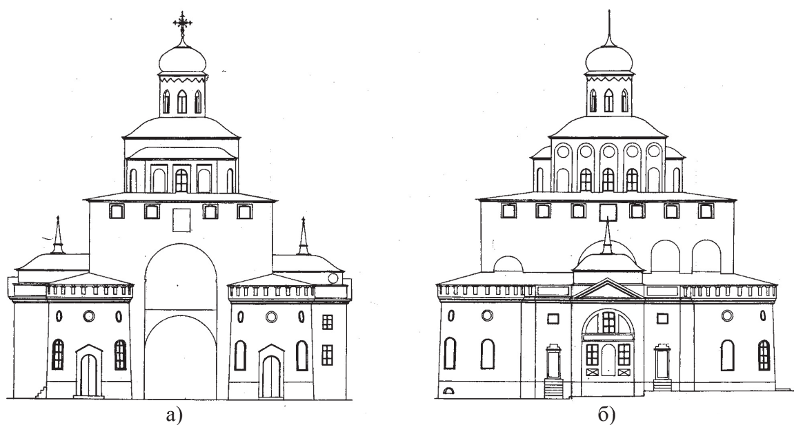
Рис. 19. Владимир. Золотые ворота. Рисунок-чертеж П.Б. Постновой а – восточный фасад; б – южный фасад
