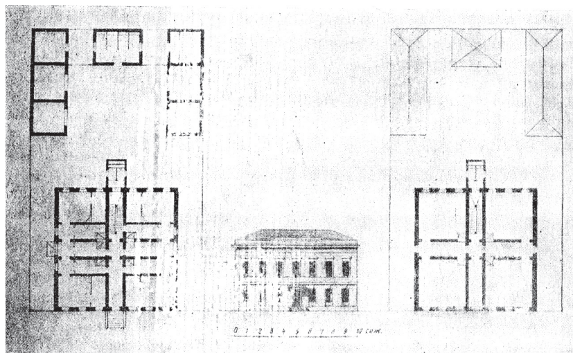
Рис. 9. Владимир. Общественные здания конца XVIII – начала XIX в.: а – фрагмент застройки Соборной площади: 1 – Дворянское собрание 1826 г.; 2 – мужская гимназия 1835 – 1841 гг.; 3 – народное училище конца XVIII в.; б – «образцовый» проект уездного училища 1830 г. [128]
