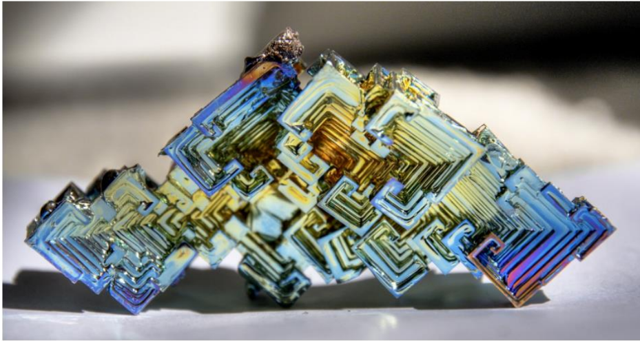
Рис. 3: Кристалл висмута.
