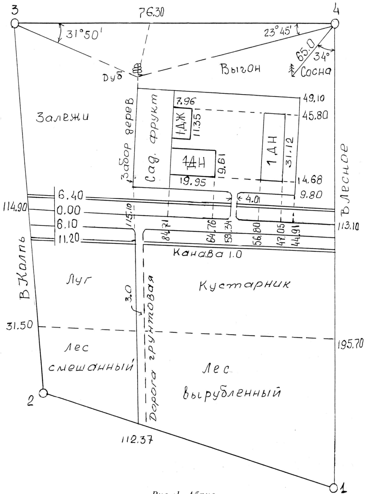
Рис. 1. Абрис
