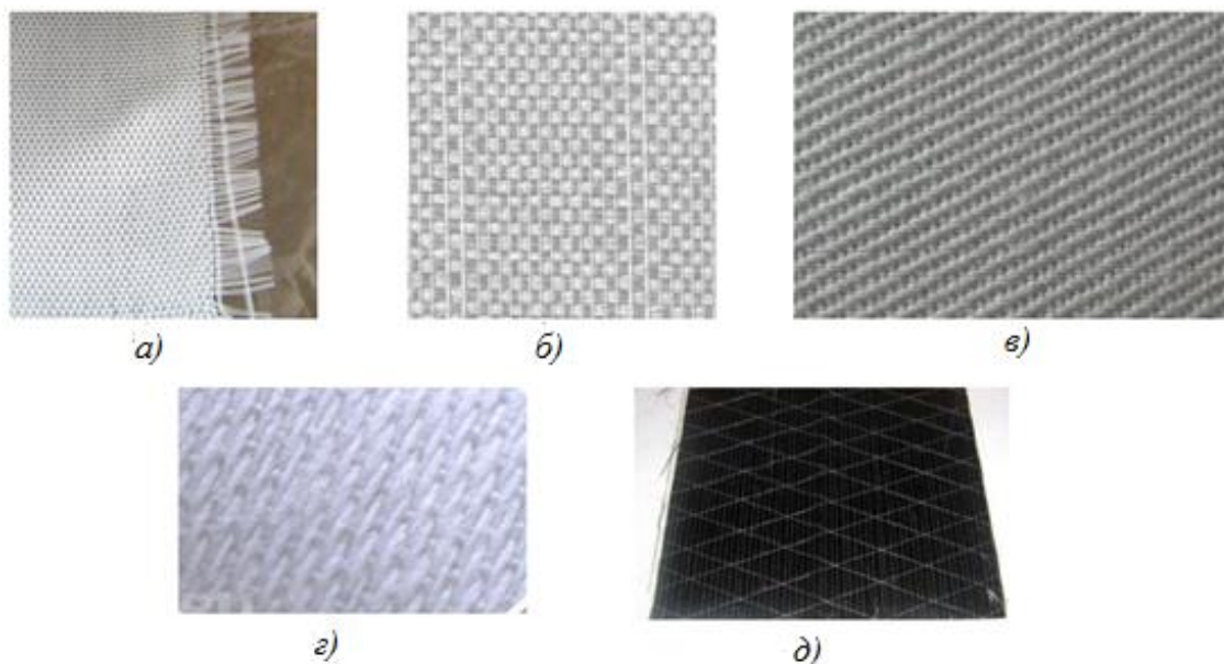
Рисунок 6.3 – Виды переплетений стеклотканей: a – полотняное; б – сеточное; в – саржевое; г – сатиновое; д – однонаправленное
