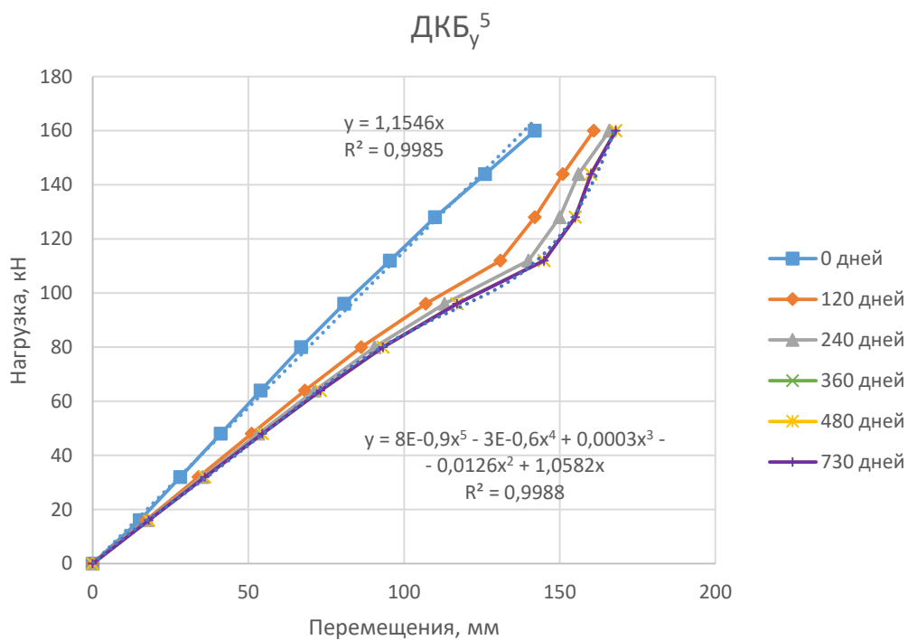
Рисунок 5.14 – Зависимость «нагрузка – перемещения» во времени ( ДКБ_y^3 , ДКБ_y^5 )
