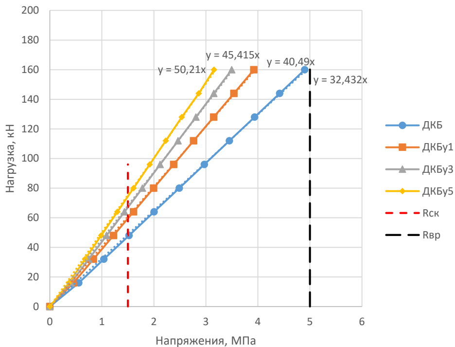
Рисунок 5.15 – Зависимость «нагрузка – касательные напряжения» для деревоклееной балки (численные исследования)
