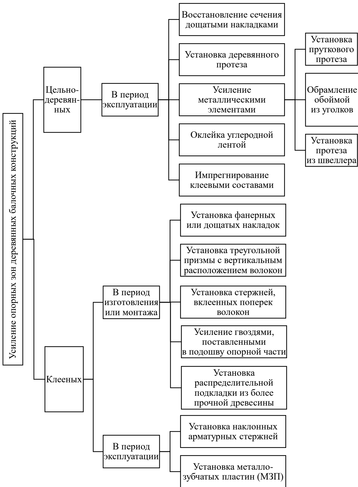
Рисунок 5.2 – Усиление опорных зон деревянных балочных конструкций
