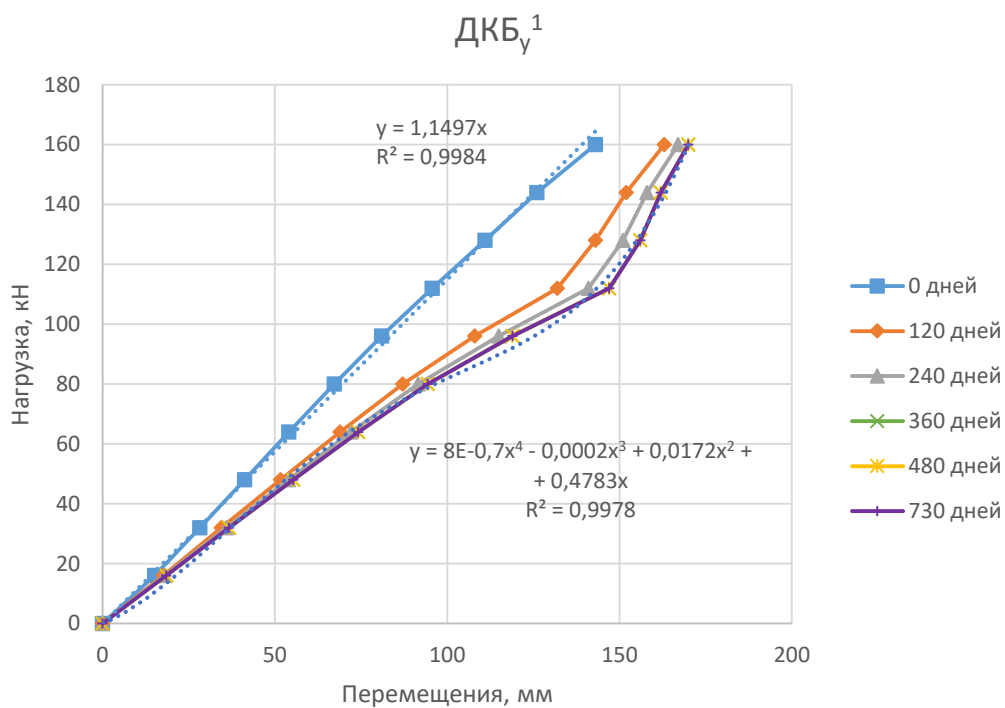
Рисунок 5.13 – Зависимость «нагрузка – перемещения» во времени (ДКБ, ДКБ y 1 )
