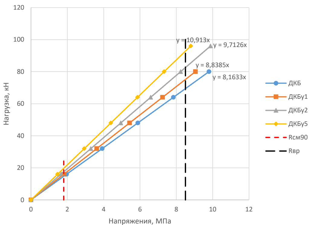
Рисунок 5.16 – Зависимость «нагрузка – сжимающие напряжения поперек волокон» для деревоклееной балки (численные исследования)
