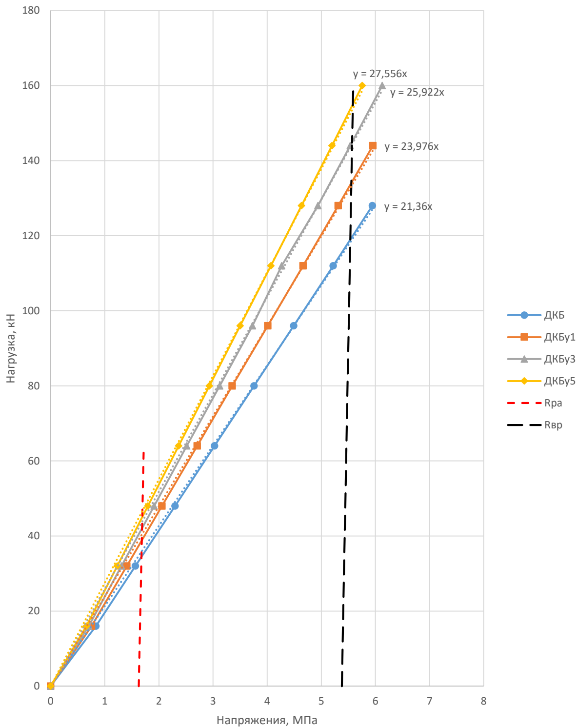
Рисунок 5.17 – Зависимость «нагрузка – растягивающие напряжения под углом к волокнам» для деревоклееной балки (угол \alpha \approx 24...25^\circ ) (численные исследования)
