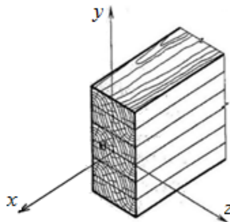
Рисунок 5.3 – Клееный пакет как трансверсально-изотропный материал
