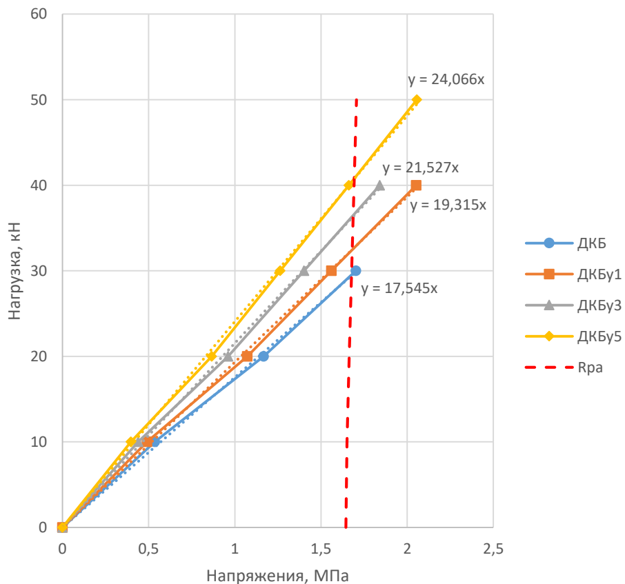
Рисунок 5.7 – Зависимость «нагрузка – растягивающие напряжения под углом к волокнам» для деревоклееной балки (угол \alpha \approx 24...25^\circ ) (инженерный расчет)
