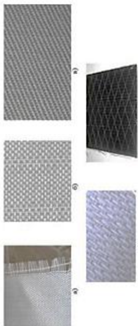
Виды переплетения стеклотканей: а – полотняное; б – сетчатое; в – саржевое; г – диагонально-решетчатое
