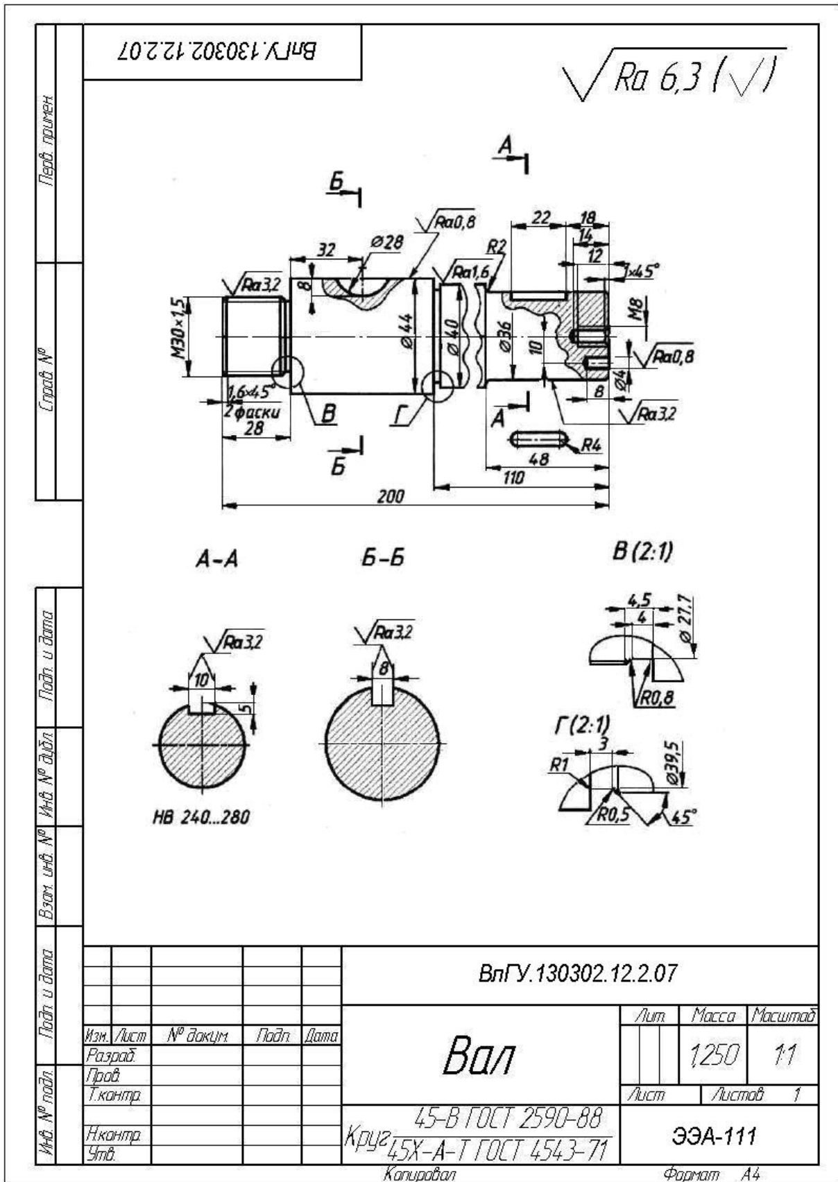
Рис. В.8 – Чертеж детали
