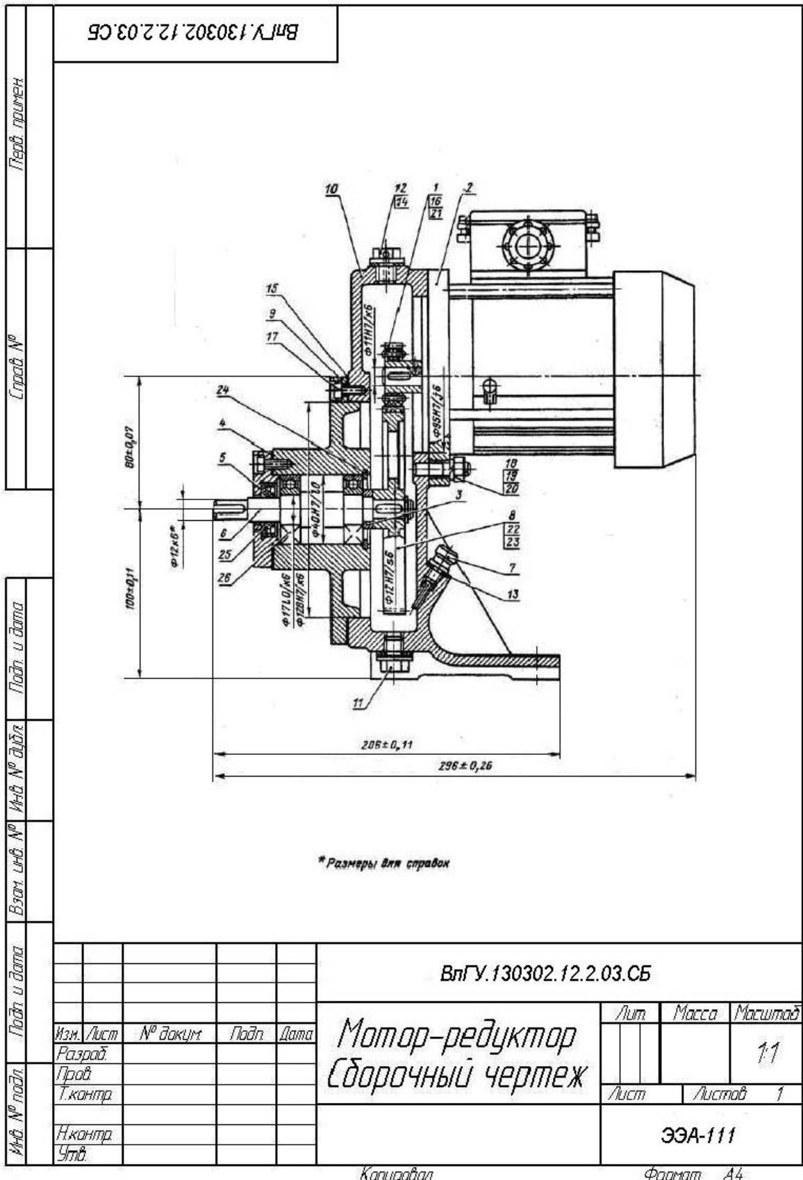
Рис. В.4 – Сборочный чертеж
