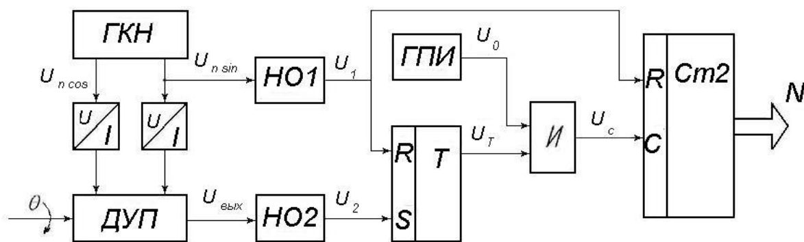
ГКН - генератор квадратурных напряжений; U/I - преобразователь напряжения в ток; НО2 - нуль орган; ГПИ - генератор прямоугольных импульсов; И - логический элемент И; Т - триггер; Cm2 - двоичный счетчик; N - цифровой код.
