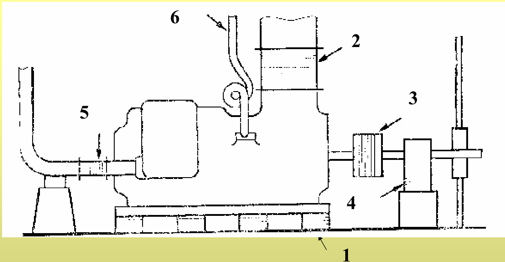
Рис. 29 Схема виброизоляции двигателя
