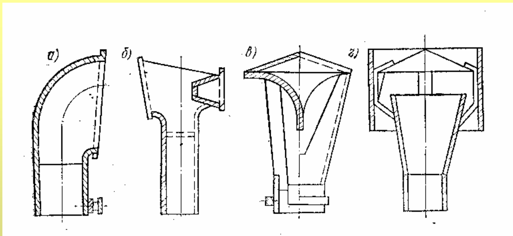
Рис. 14 Дефлекторы
