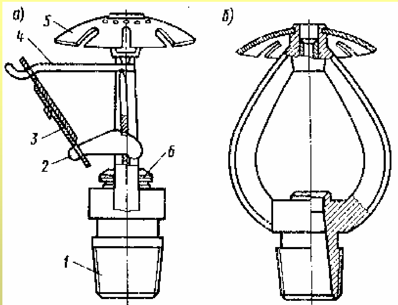
Рис. 54 Оросители - спринклерный (а) и дренчерный (б):
