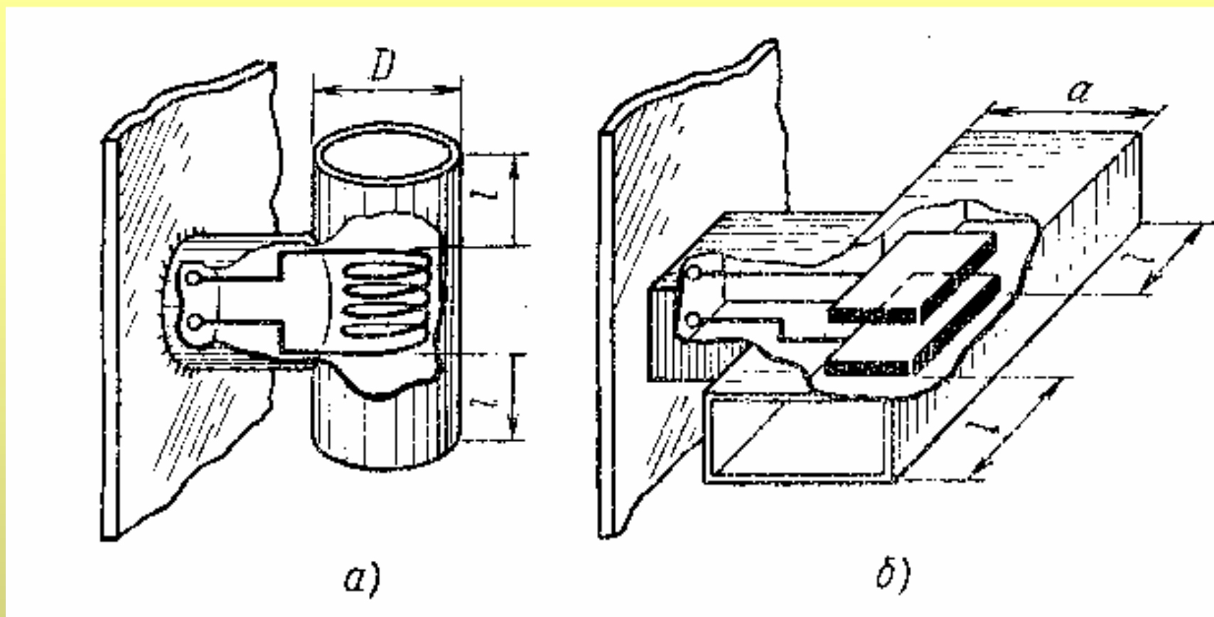
Рис. 40 Экранирование источников электромагнитных излучений.
