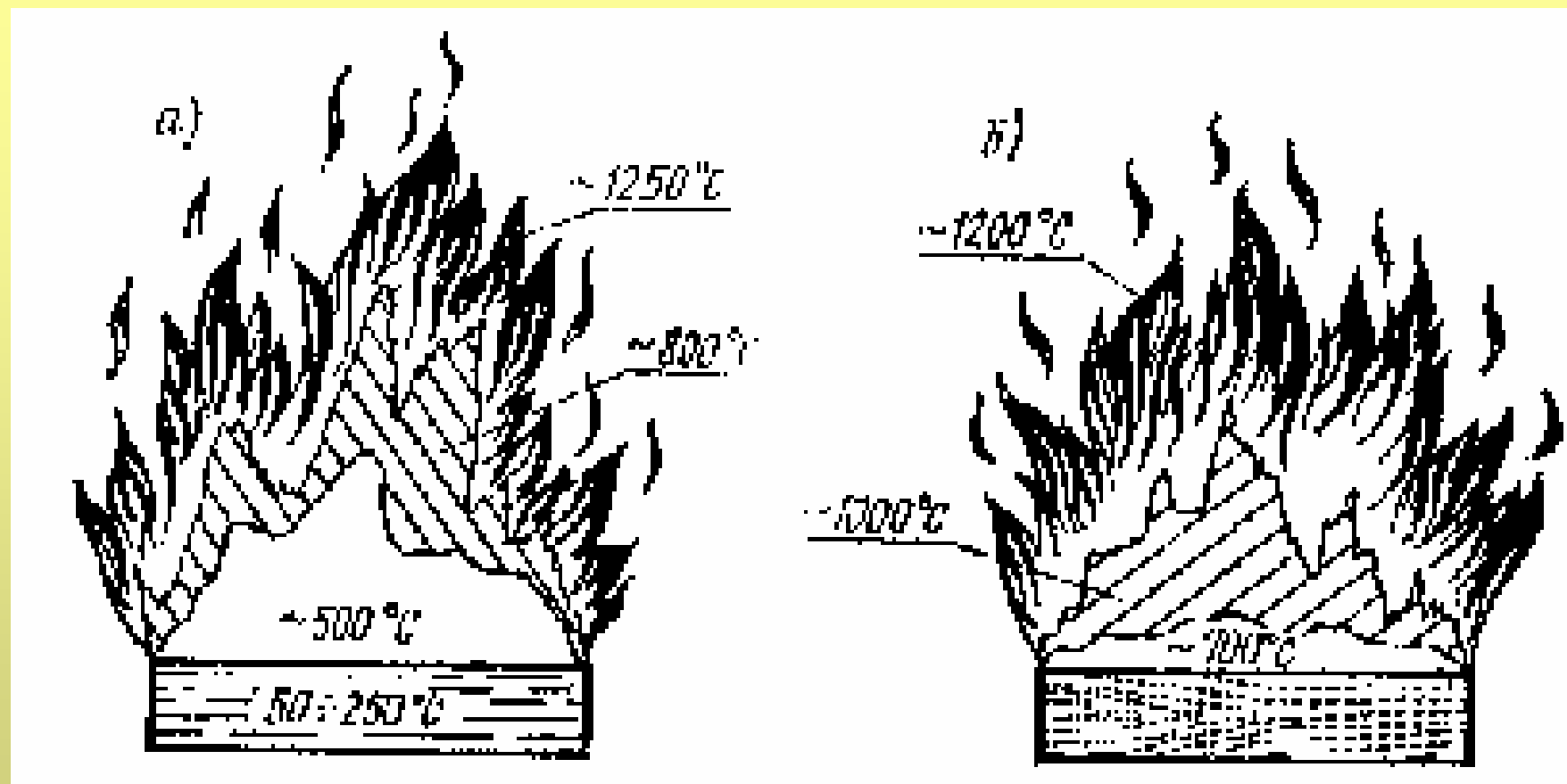
Рис. 46 Распространение температур в пламени при горении жидкостей (а) и твёрдых материалов (б)
