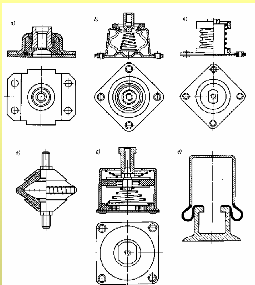
Рис. 28 Виброизоляторы
