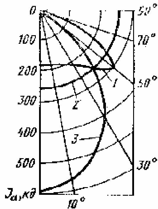
Рис. 35 Кривые силы света светильника
