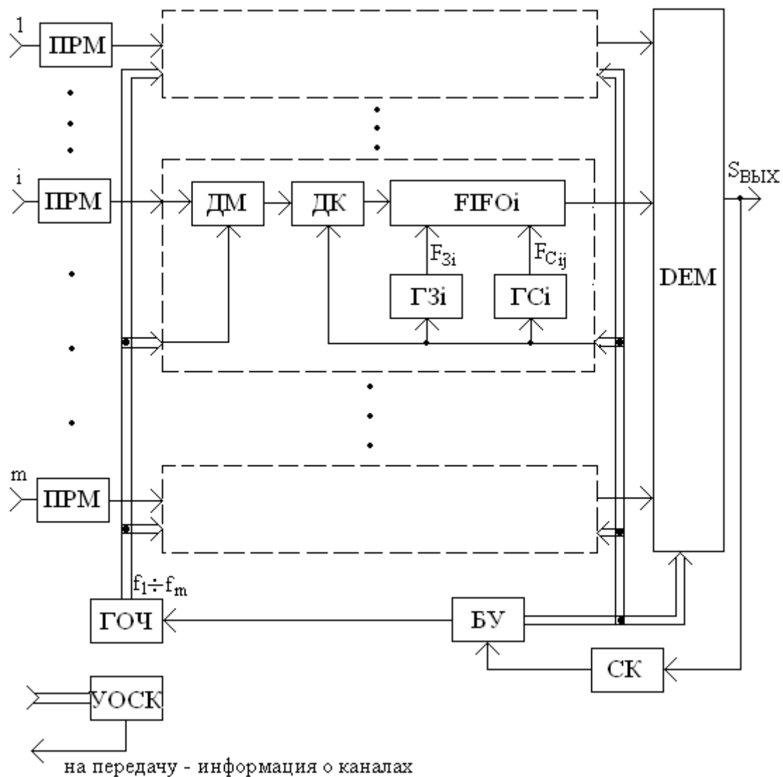
Рисунок 2 – Приемная часть системы передачи
