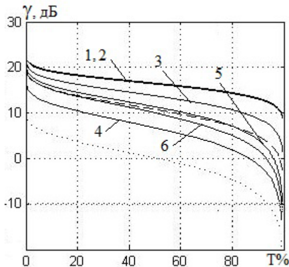
Рисунок 7 – Величина «с/п» = -10 дБ
