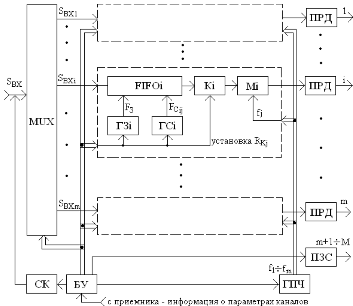
Рисунок 1 – Передающая часть системы передачи
