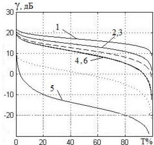
Рисунок 8 – Величина «с/п» = 10 дБ
