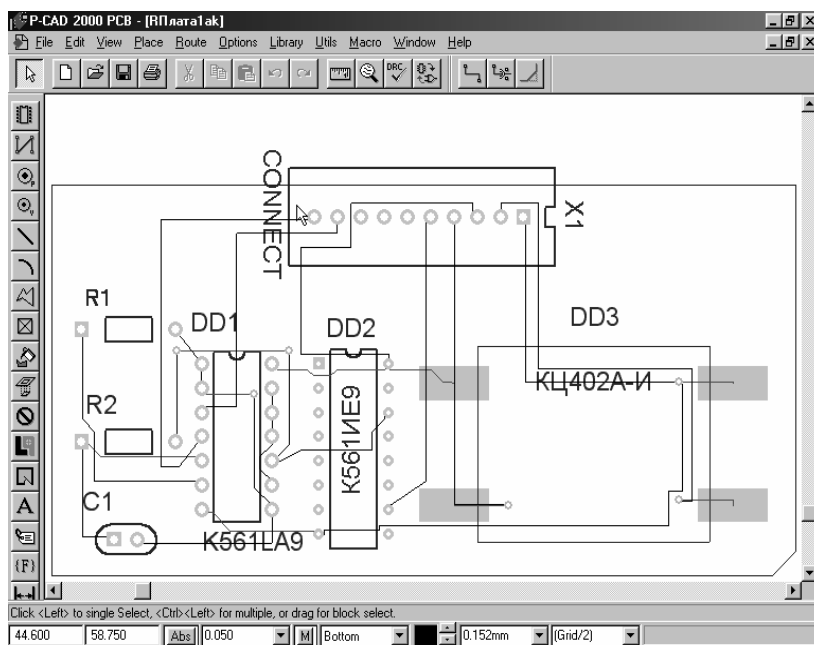
Рис. 38. Результат коррекции быстрой автотрассировки схемы
