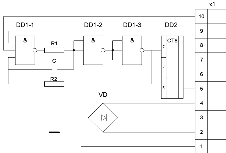
Рис. 27. Принципиальная схема генератора
