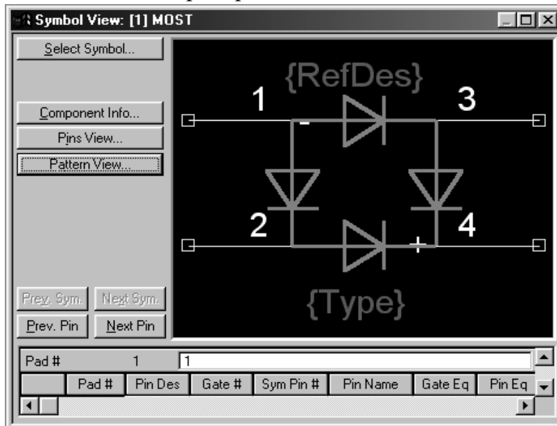
Рис. 22. Изображение символа схемы
