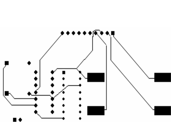
Рис. 42. Слой Top
