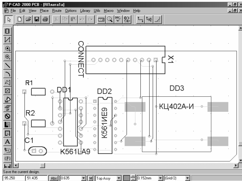
Рис. 37. Результат быстрой автотрассировки схемы
