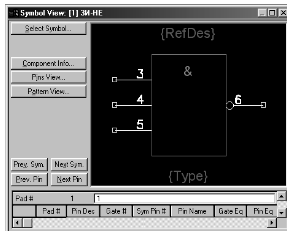
Рис. 25. Изображение символа элемента
