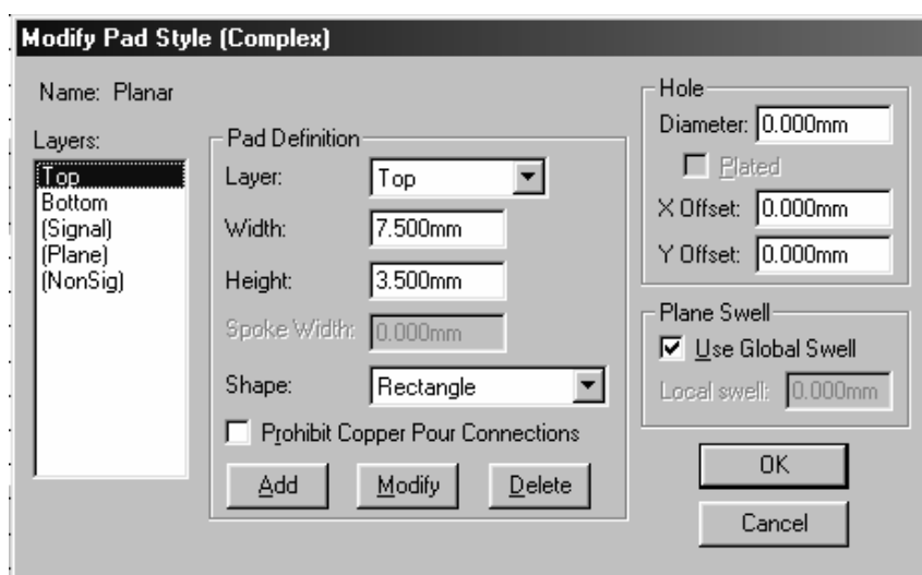
Рис. 14. Формирование контактной площадки
