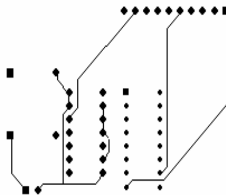
Рис. 43. Слой Bottom
