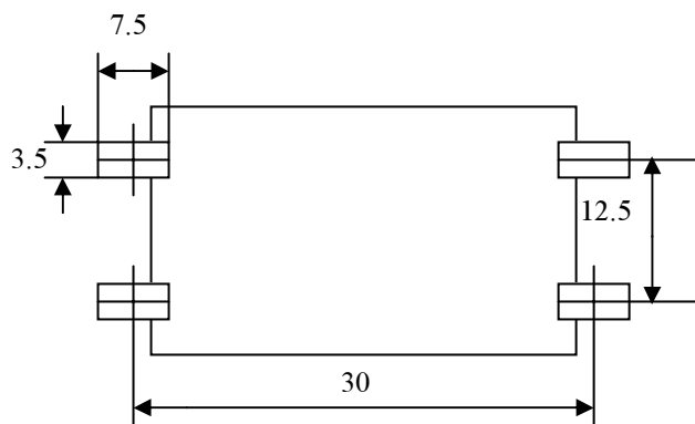
Рис. 13. Размеры посадочного места модуля КЦ402А-И
