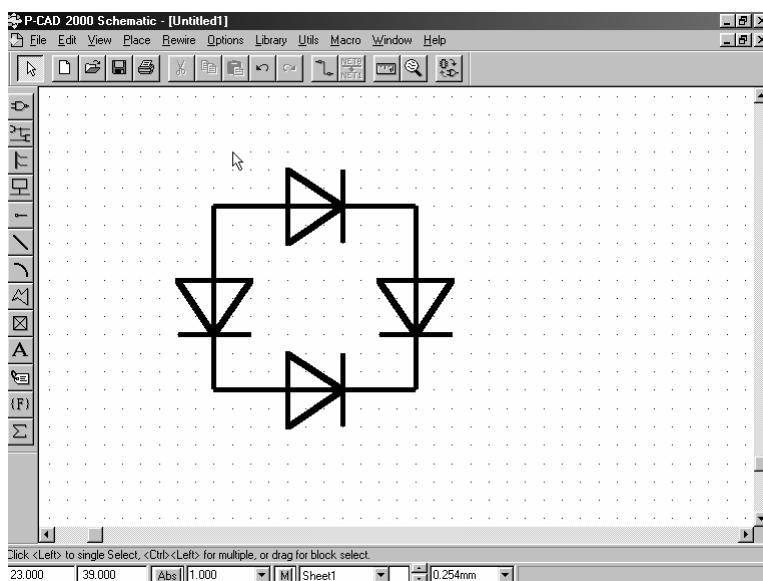
Рис. 1. Результат изображения контура символьного элемента
