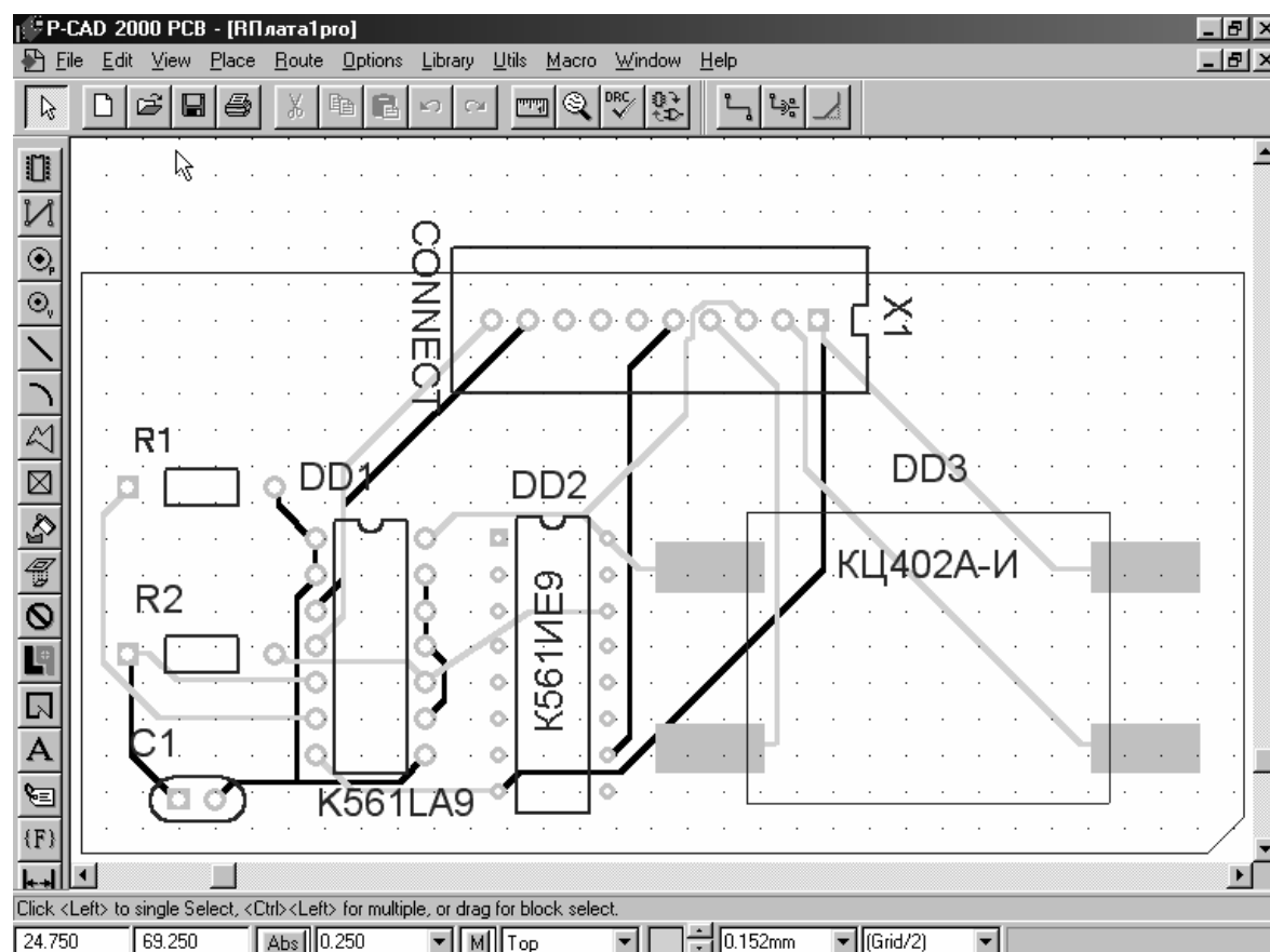
Рис. 39. Результат автотрассировки схемы с помощью профессионального трассировщика
