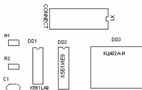
Рис. 44. Слой Top Silk
