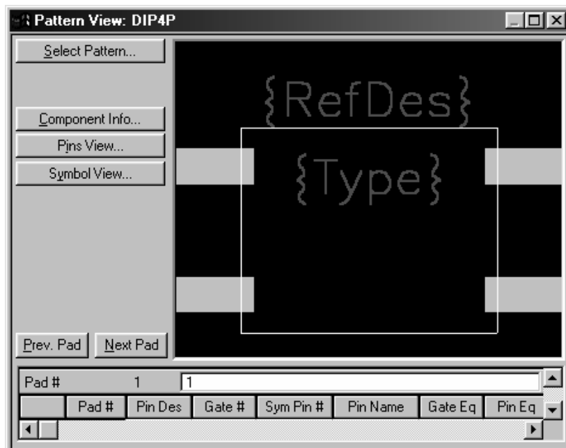
Рис. 23. Изображение посадочного места печатной платы
