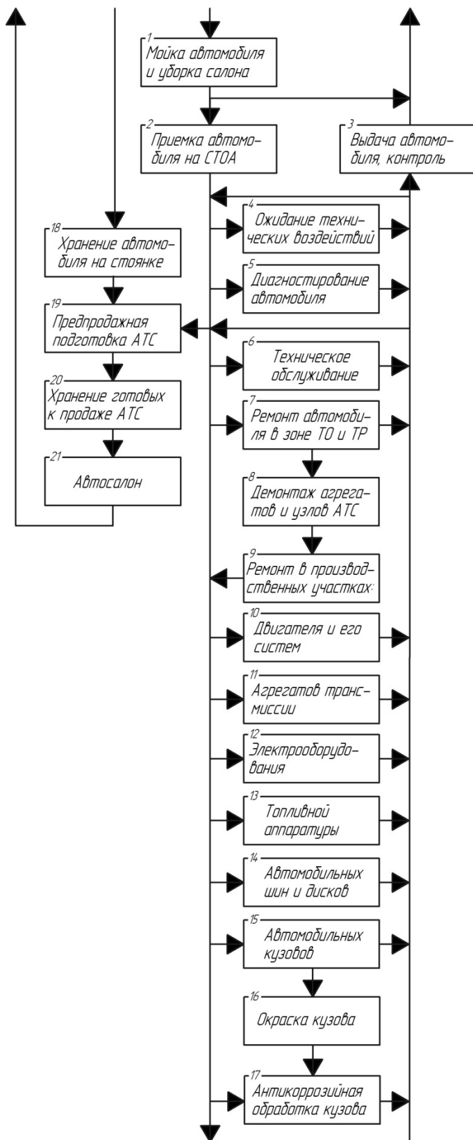
Рис. 3.5. Схема технологического процесса ТО и ТР автомобилей на СТО
