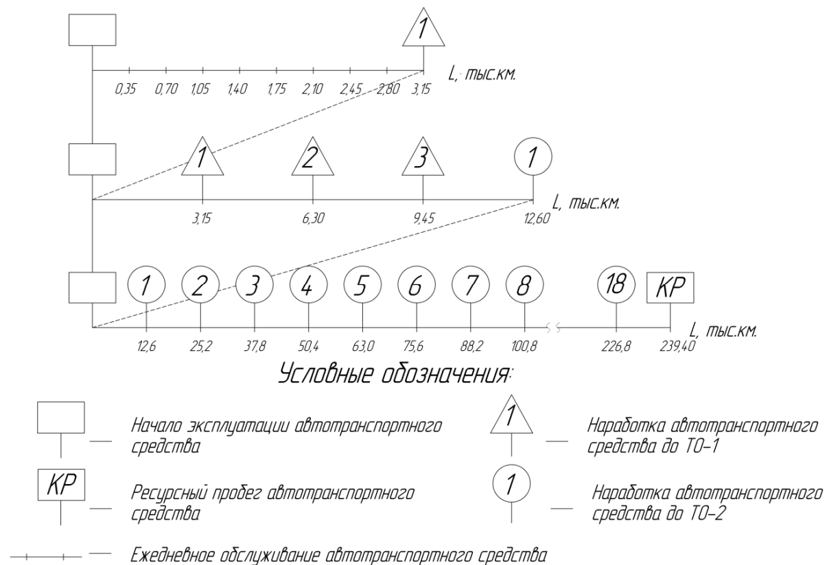
Цикловой график ТО автомобиля КамАЗ-65117
