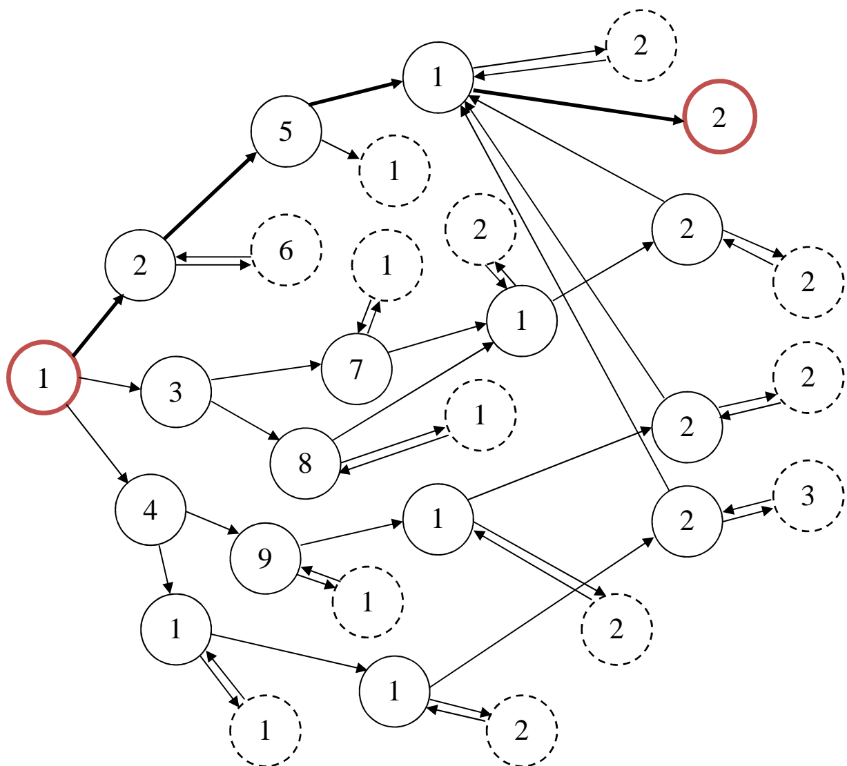
Рис. 3. Структура обучающего теста
