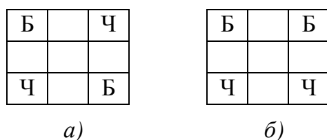
Рис. 1. Перемещение шахматных коней
