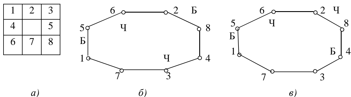
Рис. 2. Интерпретация в виде графа перемещения шахматных коней
