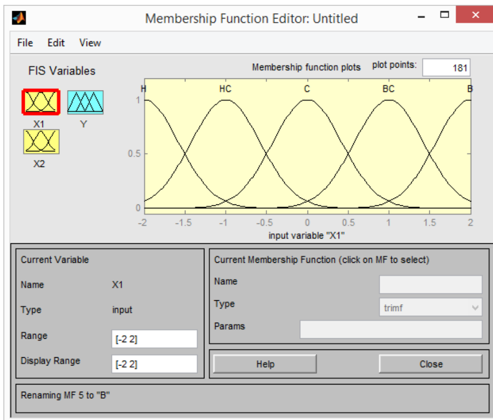
Рисунок 9. Функции принадлежности переменной x_1
