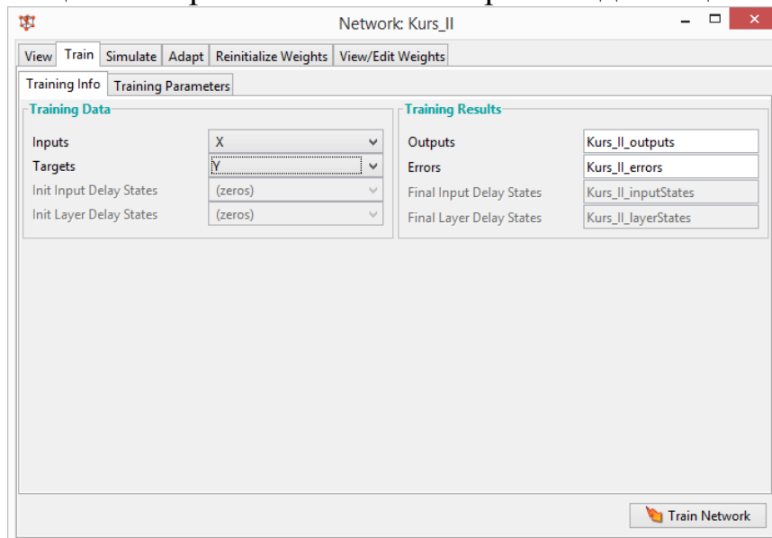
Рисунок 29. Обучение сети
