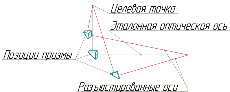
Рис. 2. – Позиции призмы при компенсации разъюстировок
