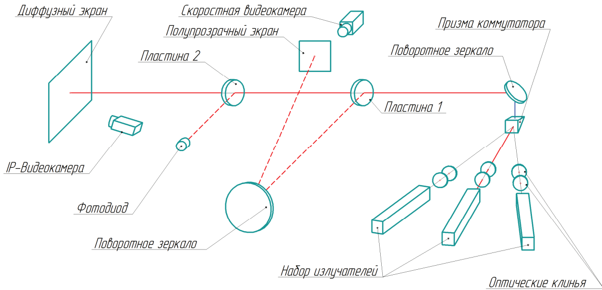
Рис. 7 – Расположение элементов оптической установки
