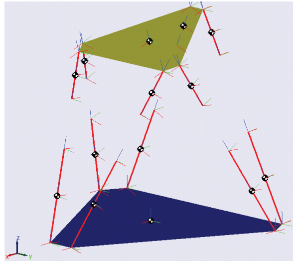
Рис. 4 – 3D-визуализация гексапода
