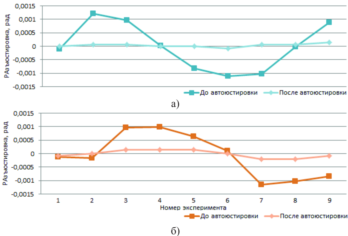
Рис. 15 – Сравнительные графики разъюстировок: а) – горизонтальная; б) – вертикальная
