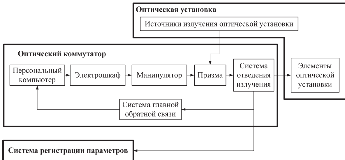
Рис. 5 – Структура оптического коммутатора
