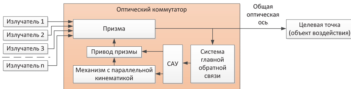
Рис. 3 – Структура разрабатываемого оптического коммутатора
