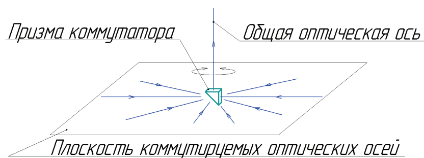
Рис. 1. – Расположение коммутируемых осей
