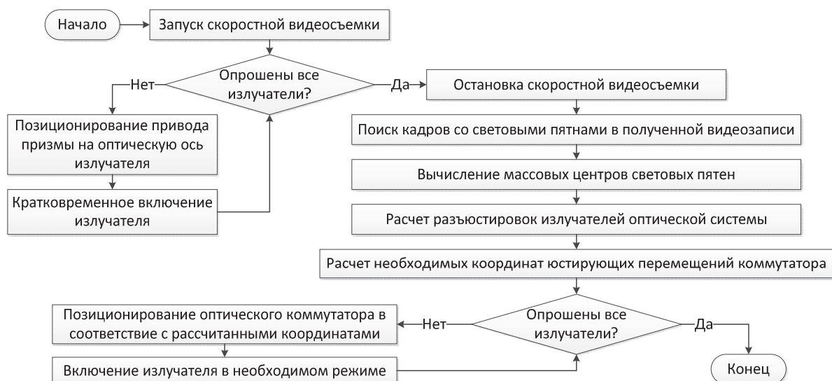
Рис. 6 – Последовательность действий коммутатора в составе оптической установки
