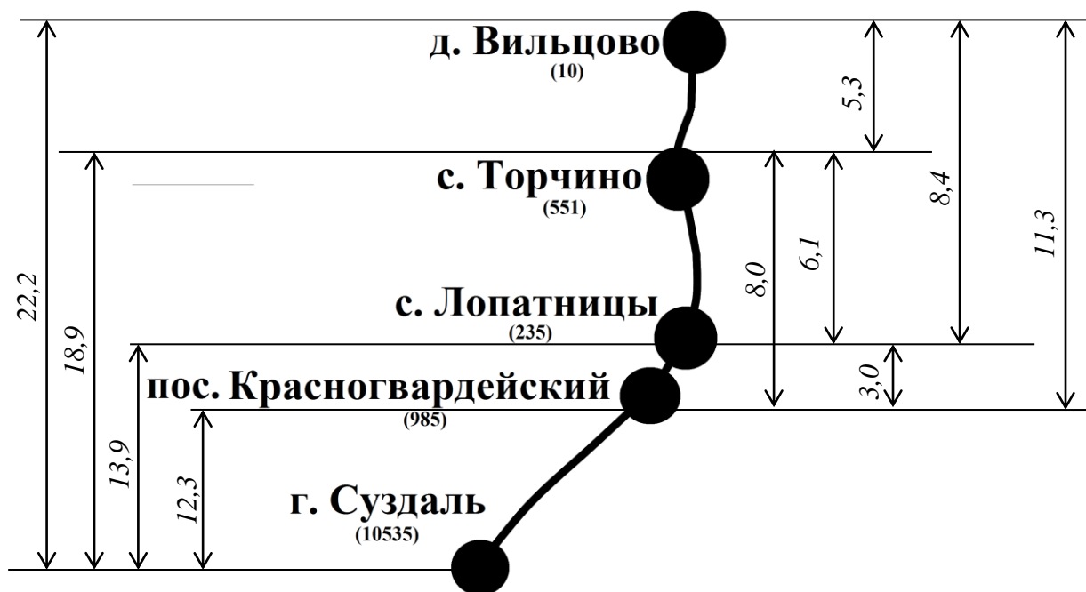
Рис. 3. Схема расположения корреспондирующих пунктов на участке федеральной трассы М-7 Владимир-Суздаль-Иваново (в скобках под населенными пунктами указано число жителей), расстояния между населенными пунктами приведены в километрах
