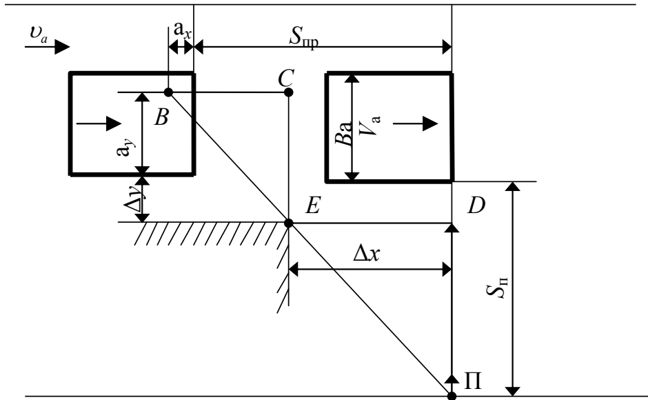
Рис. 4. Схема дорожно-транспортного происшествия: a_x – расстояние от водителя до передней части автомобиля; a_y – расстояние от водителя до боковой стороны автомобиля; \Delta x – расстояние между линией следования пешехода и предметом, ограничивающим обзорность; \Delta y – расстояние между автомобилем и предметом, ограничивающим обзорность; S_{пр} – приближение автомобиля к месту наезда; B_a – габаритная ширина автомобиля; v_a – скорость автомобиля; S_{\Pi} – путь, пройденный пешеходом, до наезда на него автомобиля; B – точка расположения водителя; \Pi – пешеход; E – вершина угла предмета, ограничивающего обзорность
