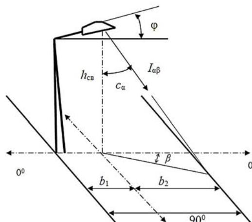
Рис. 2. Схема расчета углов при расположении светильника РКУ 01-250-011 над освещаемой полосой
