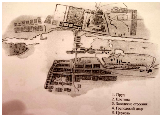
Генеральный план Гусевского металлургического завода начала XIX в. Фото из статьи Г. С. Цыганкина «Основные структурообразующие элементы заводской усадьбы Замосковского горного округа XVIII – первой половины XIX в.»
