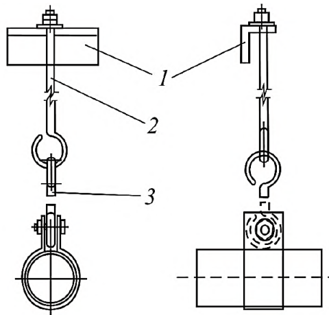
Рис. 7.18. Подвесная опора:
