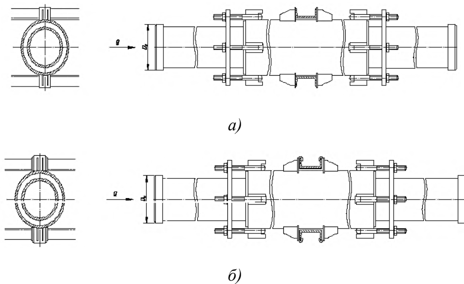
Рис. 7.19. Опоры неподвижные лобовые для сальниковых компенсаторов
