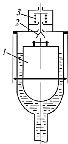
Рис. 3.1. Воздухоотводчик:
