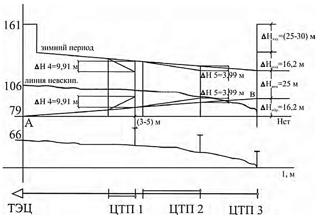
Рис. 8.5. Пьезометрический график участка трубопровода от ТЭЦ до ЦТП 3
