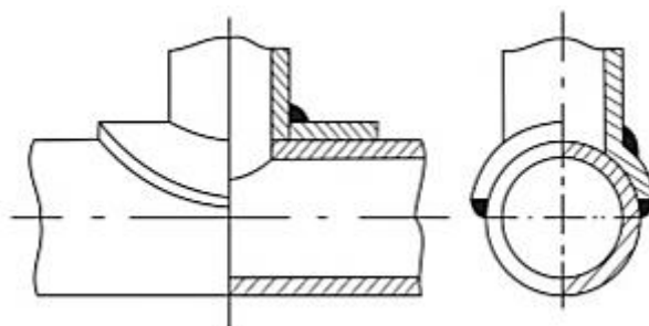
Рис. 7.5 Врезка с накладным воротником
