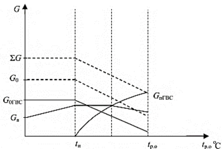
Рис. 4.9. График суммарного расхода сетевой воды в открытых водяных системах
