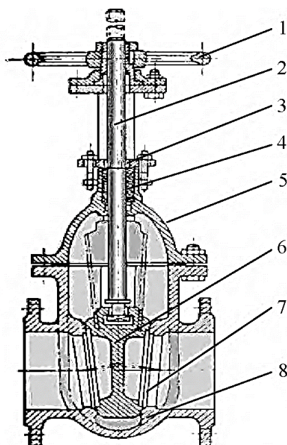
Рис. 7.15. Задвижка клиновая с цельным клином:
