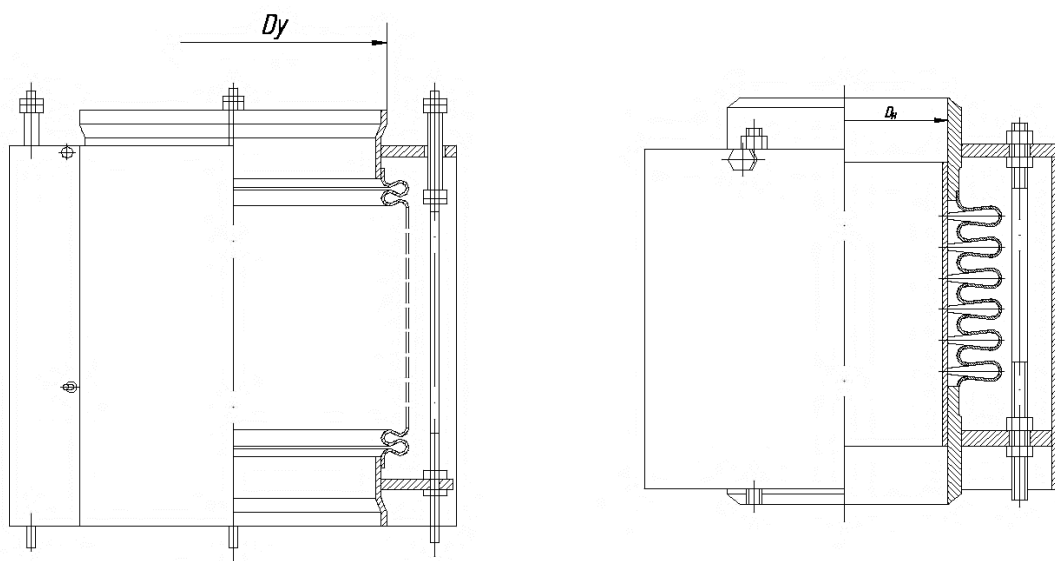
Рис. 7.24. Осевые сильфонные компенсаторы
