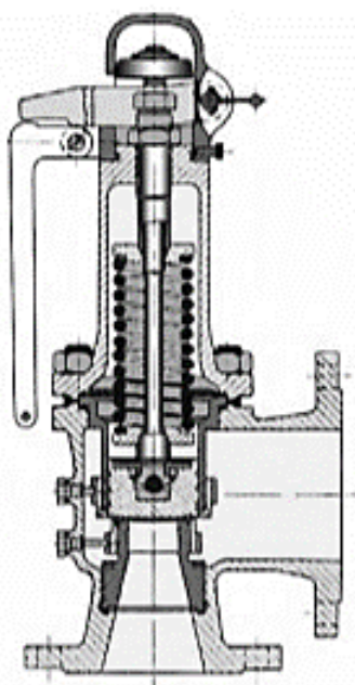
Рис.76.11. Пружинный клапан
