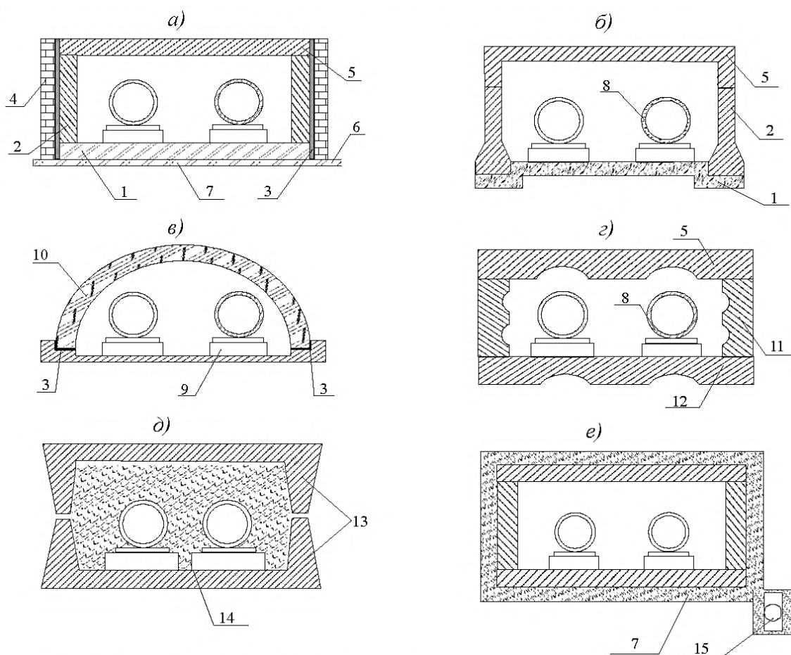
Рис. 8.2. Непроходимо каналы:
