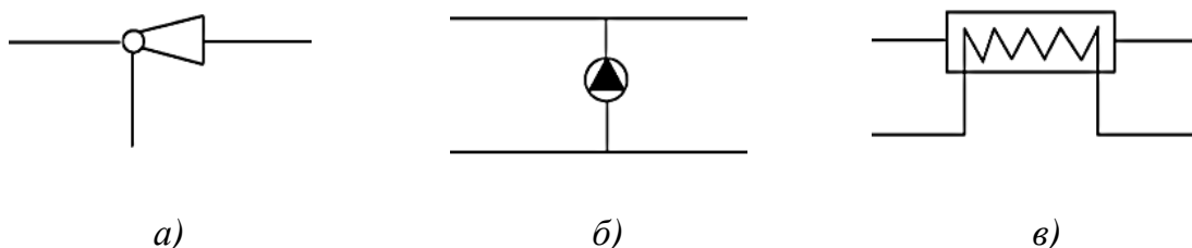
Рис. 2.5. Присоединения со снижением потенциала: а – элеваторные; б – насосные; в – теплообменник
