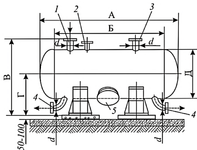
Рис. 3.9. Установка цилиндрического аккумулятора теплосети по полу:
