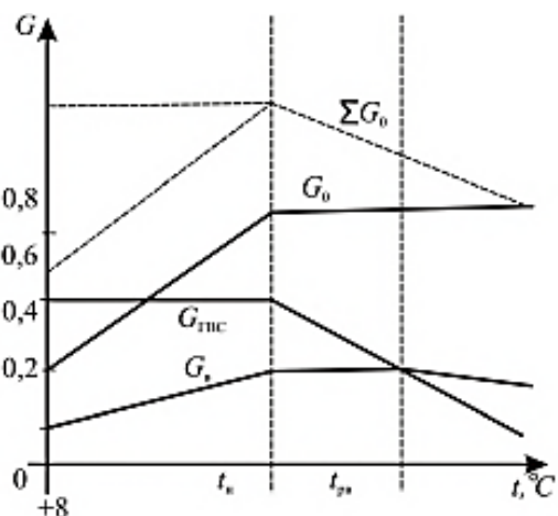
Рис. 4.8. График суммарного расхода сетевой воды в закрытых водяных системах
