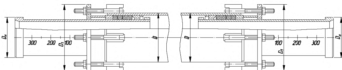
Рис. 7.26. Сальниковый компенсатор двухсторонний
