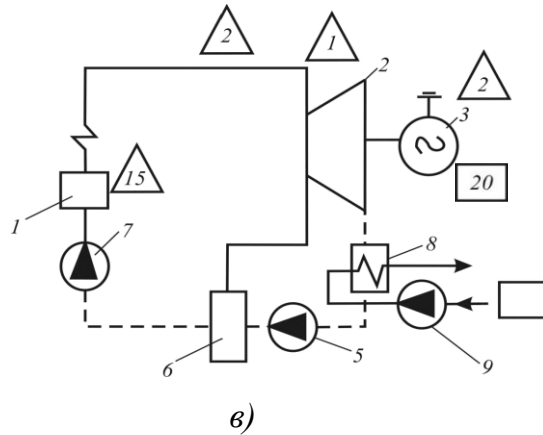
Рис. 1.1. Принципиальные схемы отдельного и комбинированного процессов выработки тепла и электроэнергии (окончание): а – отдельный процесс (КЭС); б – отдельный процесс (РК); в – комбинированный процесс (ТЭЦ); 1 – котел; 2 – турбина; 3 – генератор; 4 – конденсатор; 5 – конденсаторный насос; 6 – регенеративный подогреватель; 7 – питательный насос; 8 – подогреватель сетевой воды; 9 – сетевой насос; \tau – потери тепла, %; \Delta – полезно используемое тепло, %
