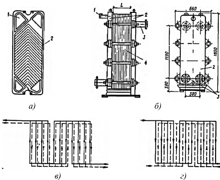
Рис. 2.7. Пластинчатый водоподогреватель:
