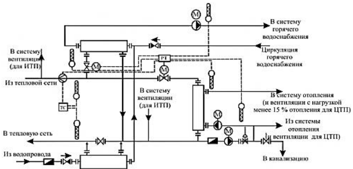
Рис. 5.1. Двухступенчатая схема присоединения водоподогревателей горячего водоснабжения в ИТП с водоструйным элеватором и автоматическим регулированием расхода теплоты на отопление
