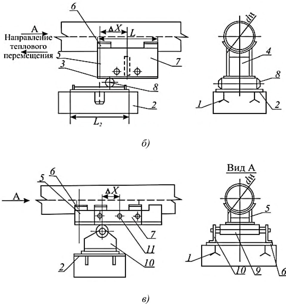
Рис. 7.17. Опоры подвижные (продолжение)
