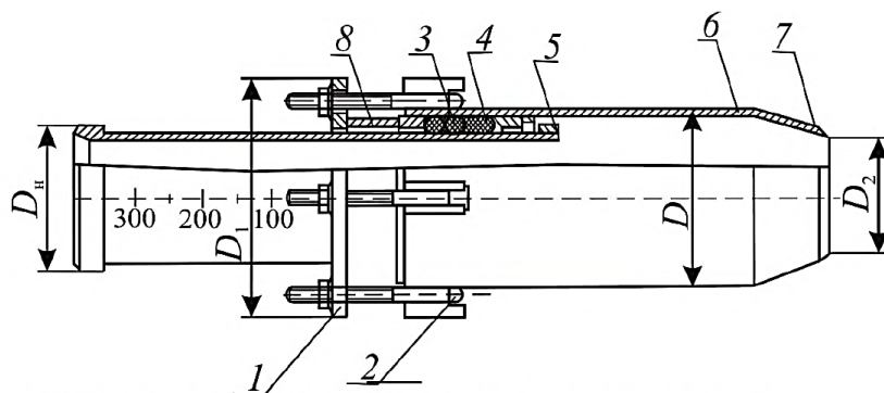
Рис. 7.25. Сальниковый компенсатор односторонний: 1 – нажимной фланец; 2 – болтовое соединение; 3 – сальниковая набивка; 4 – контр-букса; 5 – стакан; 6 – корпус; 7 – переход диаметра; 8 – грунт букса
