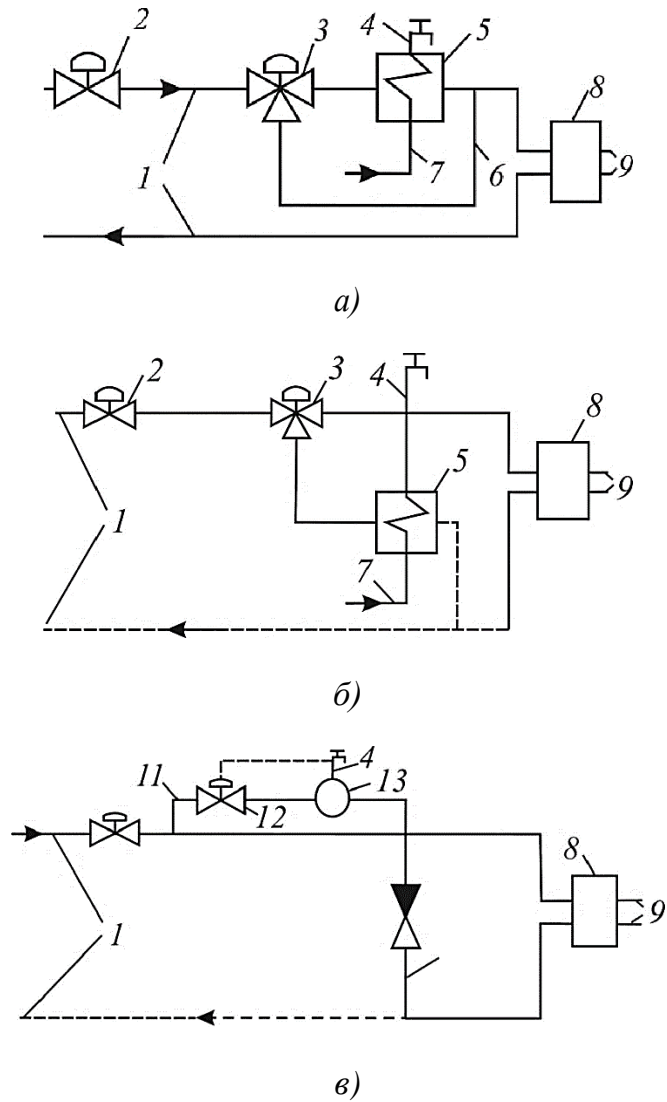
Рис. 4.1 Схемы абонентских вводов связанной подачи тепла в систему отопления:
