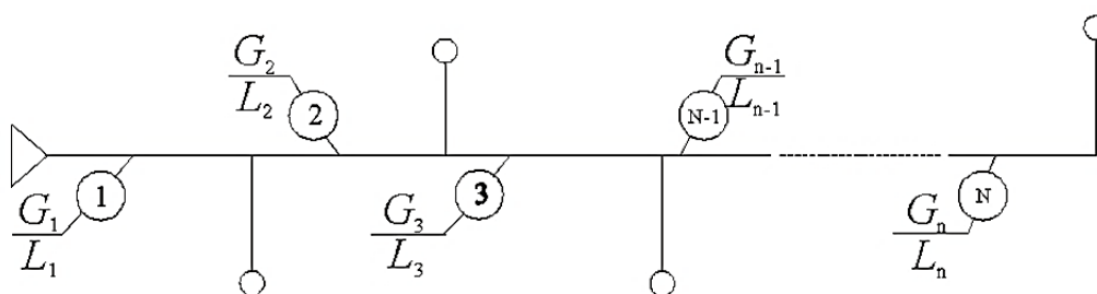
Рис. 8.3. Расчетная схема тепловой сети
