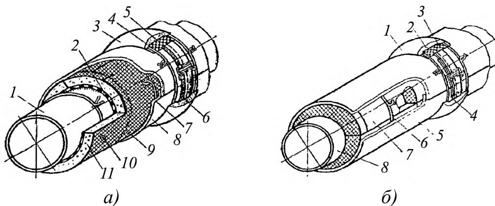
Рис. 9.1. Изоляция трубопроводов:
