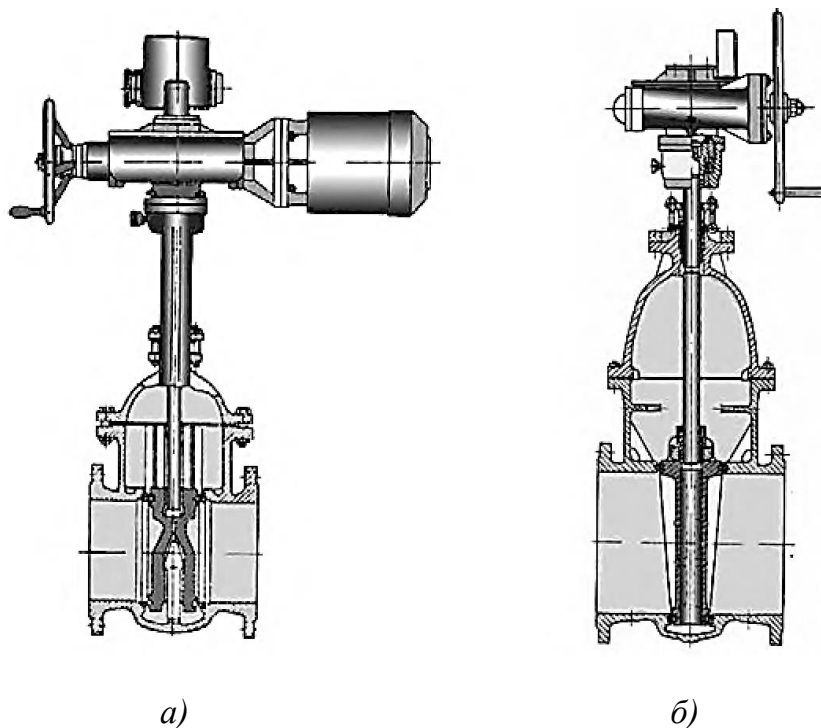
Рис. 7.16. Задвижка: а – параллельная с выдвижным шпинделем и электроприводом; б – клиновая с червячным приводом
