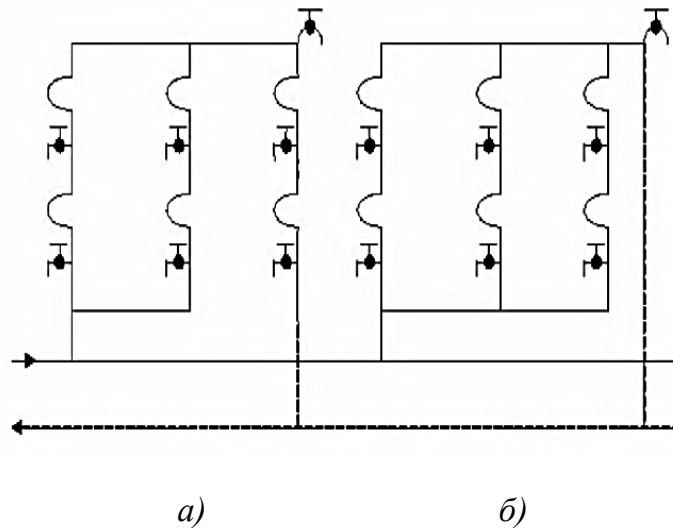
Рис. 3.6. Потенциальные закольцованные стояки: а – с водоразборным циркуляционным стояком; б – с дополнительным циркуляционным стояком
