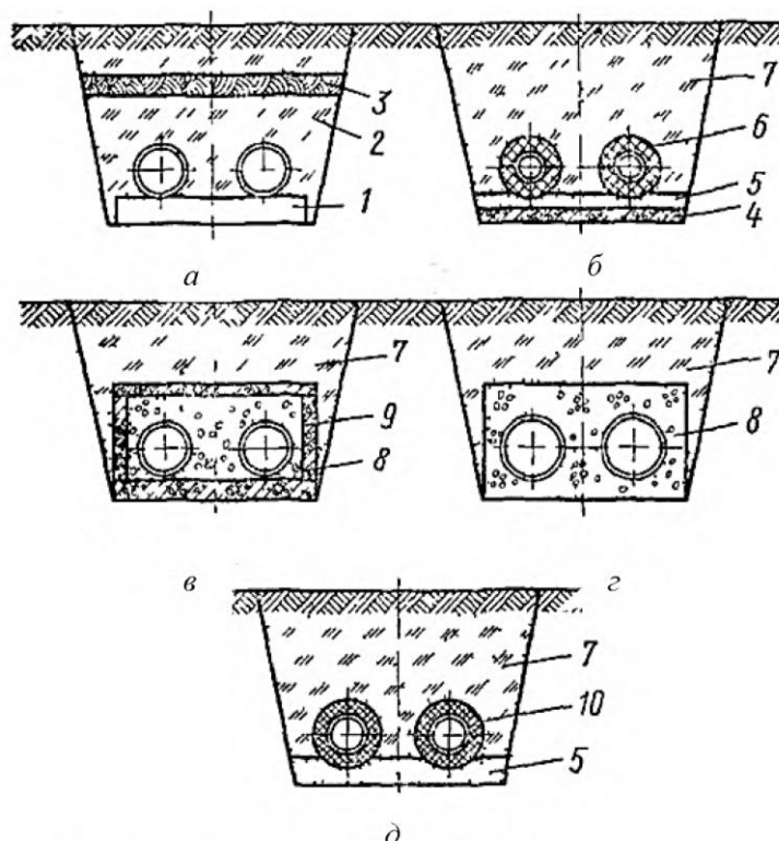
Рис. 8.3. Типы бесканальных прокладок:
