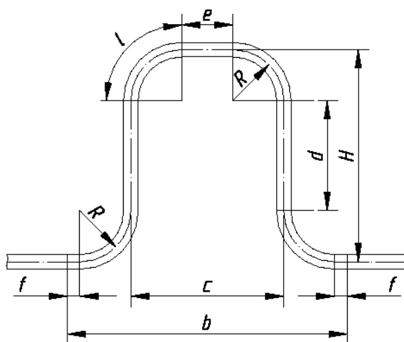
Рис. 7.27. П-образный компенсатор
