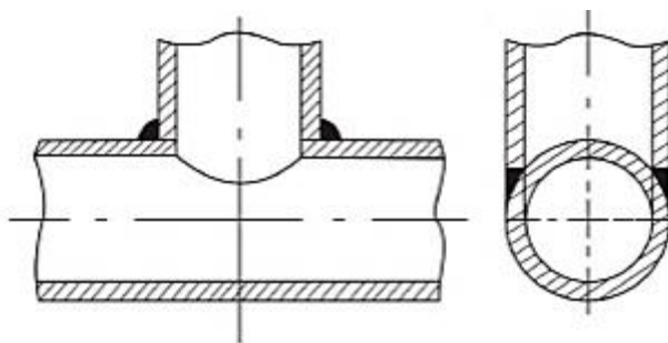
Рис. 7.4. Врезки без укрепляющих элементов
