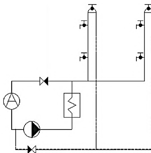
Рис. 3.8. Схема включения закрытого бака-аккумулятора
