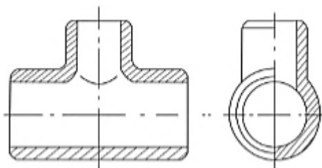
Рис. 7.6. Штампованный тройник
