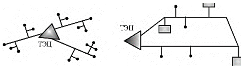
Рис. 8.2. Разновидности схем тепловых сетей: а – радиальная; б – кольцевая
