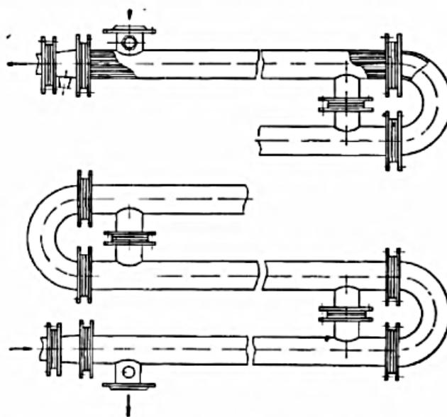
Рис. 2.6. Водно-водяной скоростной секционный подогреватель
