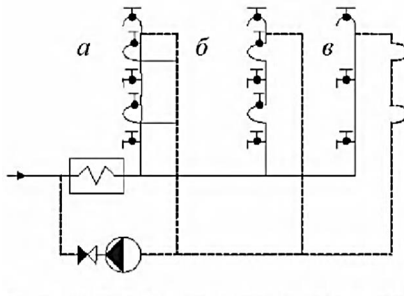
Рис. 3.4. Схема водоразборных узлов с различным присоединением полотенцесушителей к стоякам:
