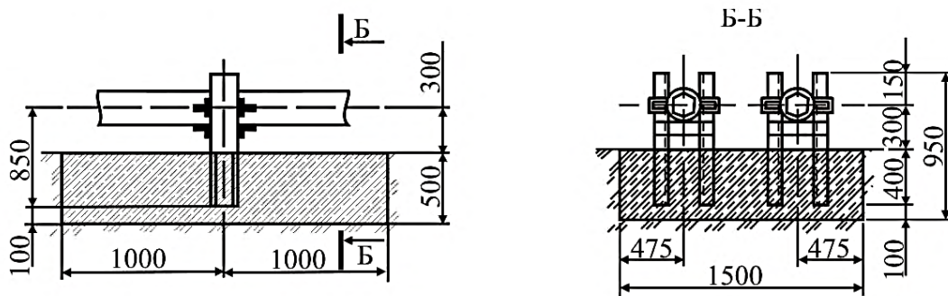
Рис. 7.22. Неподвижная отдельно стоящая опора для труб D_y 80-200 мм (подвальная)
