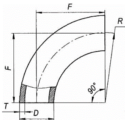
Рис. 7.2. Отвод крутоизогнутый, угол 90^\circ
