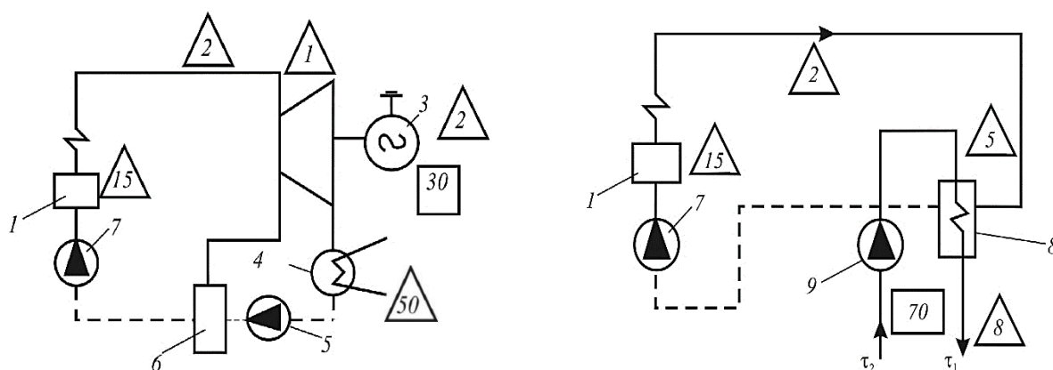
Рис. 1.1. Принципиальные схемы отдельного и комбинированного процессов выработки тепла и электроэнергии (начало)
