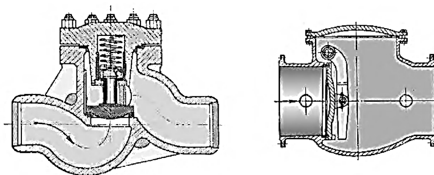
Рис. 7.13. Пружинный клапан
