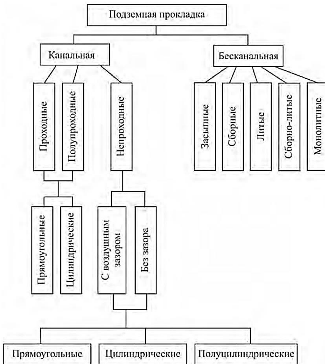
Рис. 7.28. Схема видов подземной прокладки трубопроводов
