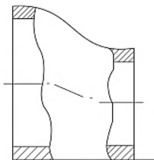
Рис. 7.9. Бесшовный эксцентрический переход трубопроводов
