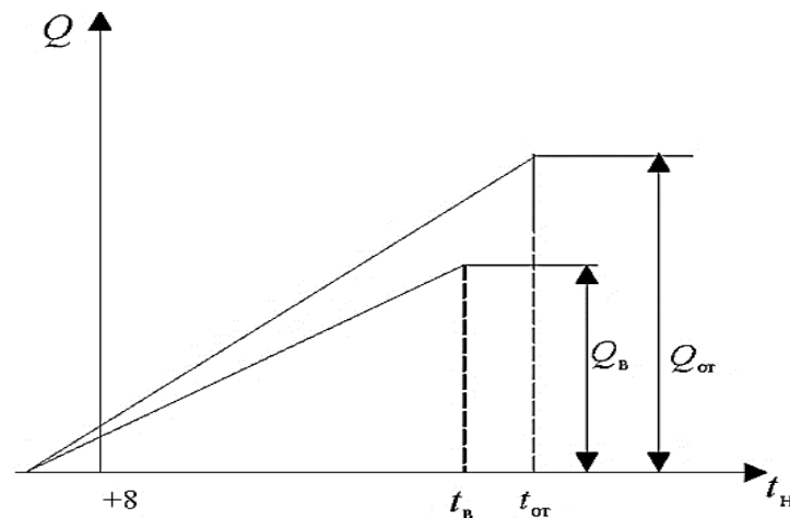
Рис. 2.1. График расхода тепла на отопление и вентиляцию
