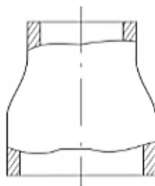
Рис. 7.8. Бесшовный концентрический переход трубопроводов
