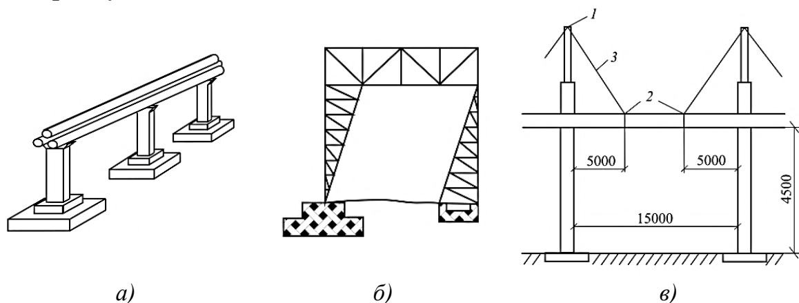
Рис. 8.4. Основные виды надземной прокладки трубопроводов: а – на отдельно стоящих опорах; б – на эстакадах; в – на подвесных (вантовых) конструкциях; 1 – металлическая вершина; 2 – подвесная опора; 3 – тяги
