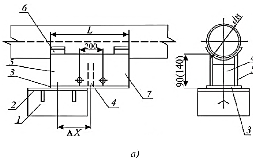
Рис. 7.17 Опоры подвижные
