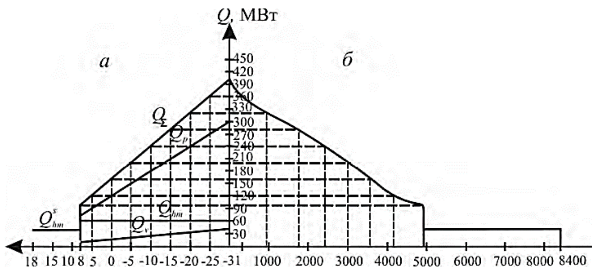
Рис.2.3. Годовой график расхода тепла
