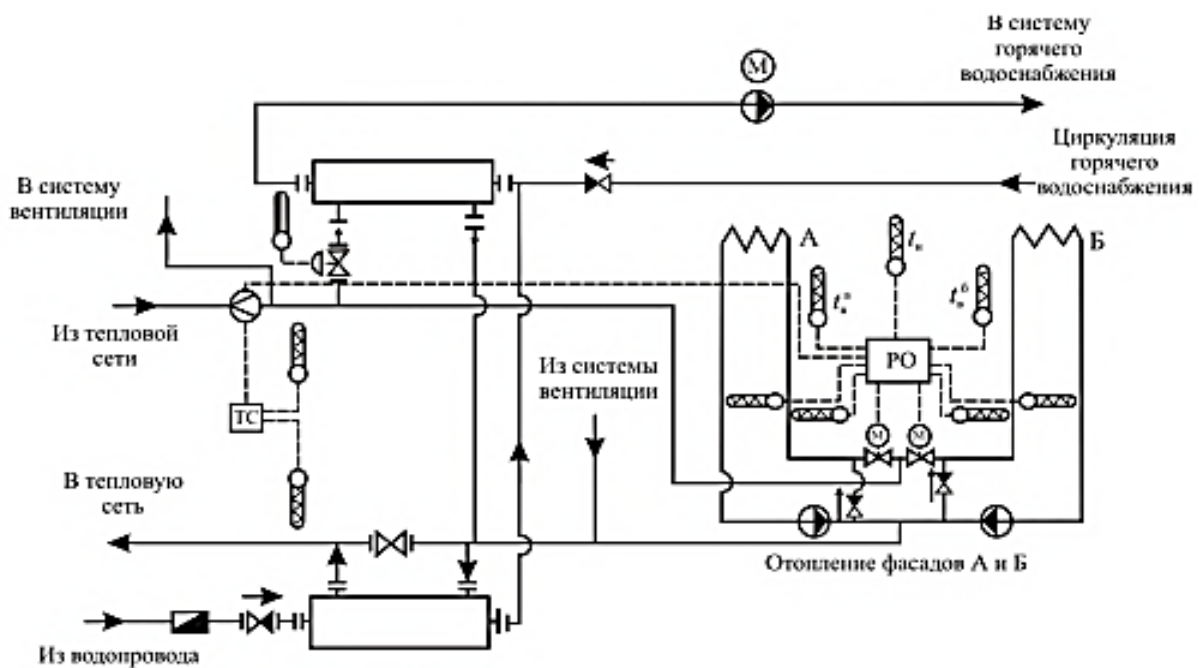
Рис. 5.2. Двухступенчатая схема присоединения водоподогревателей горячего водоснабжения с зависимым присоединением систем отопления при отсутствии регуляторов расхода теплоты на отопление в ЦТП и ИТП
