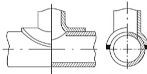
Рис. 7.7. Накладные седловины
