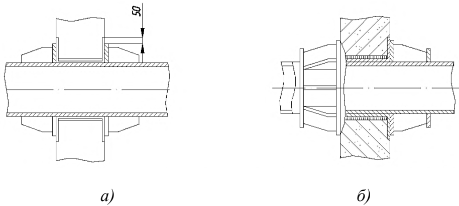
Рис. 7.21. Опоры неподвижные щитовы для трубопроводов D_H 108-1420 мм с защитой от электрокоррозии: а - обыкновенные; б - усиленные
