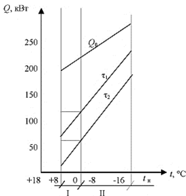
Рис. 4.3. График температур, расходов тепла и сетевой воды при комбинированном регулировании отопительной нагрузки:
