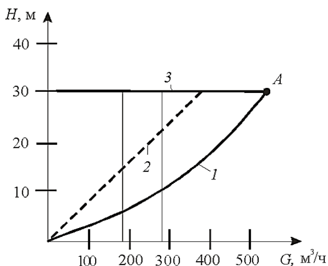
Рис. 6.1. Характеристики тепловой сети с насосами:
