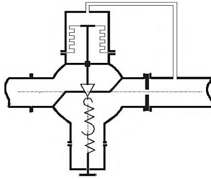
Рис. 5.5. Схема регулятора давления «до себя»
