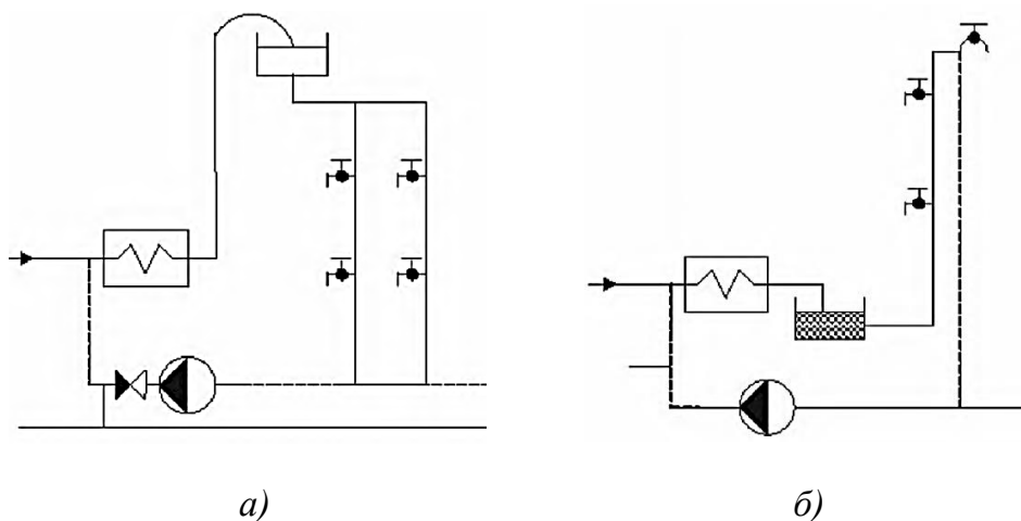
Рис. 3.7. Схема включения открытых баков-аккумуляторов: а – верхний; б – нижний
