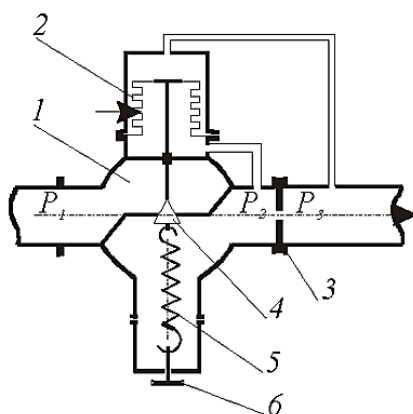
Рис. 5.4. Схема регулятора расхода (PP) прямого действия 1 – корпус; 2 – сильфон; 3 – диафрагма; 4 – односедельный клапан; 5 – пружина; 6 – натяжной винт
