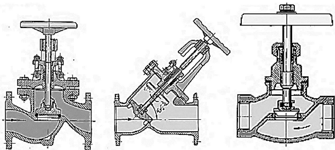
Рис. 7.14. Вентили
