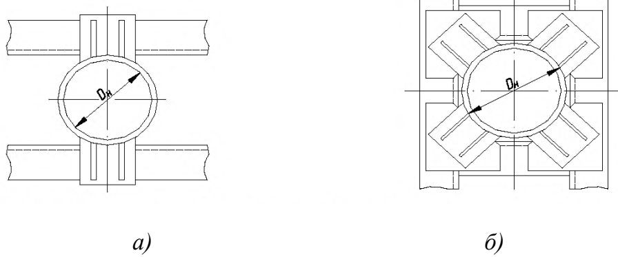
Рис. 7.20. Опоры неподвижные лобовые: а - двухпортовые для трубопроводов D_H 108-1420 мм; б - четырехпортовые для трубопроводов D_H 133-1420 мм
