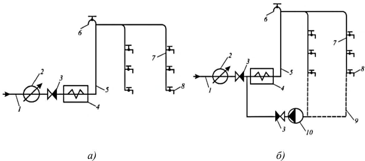
Рис. 3.2. Схема систем горячего водоснабжения:
