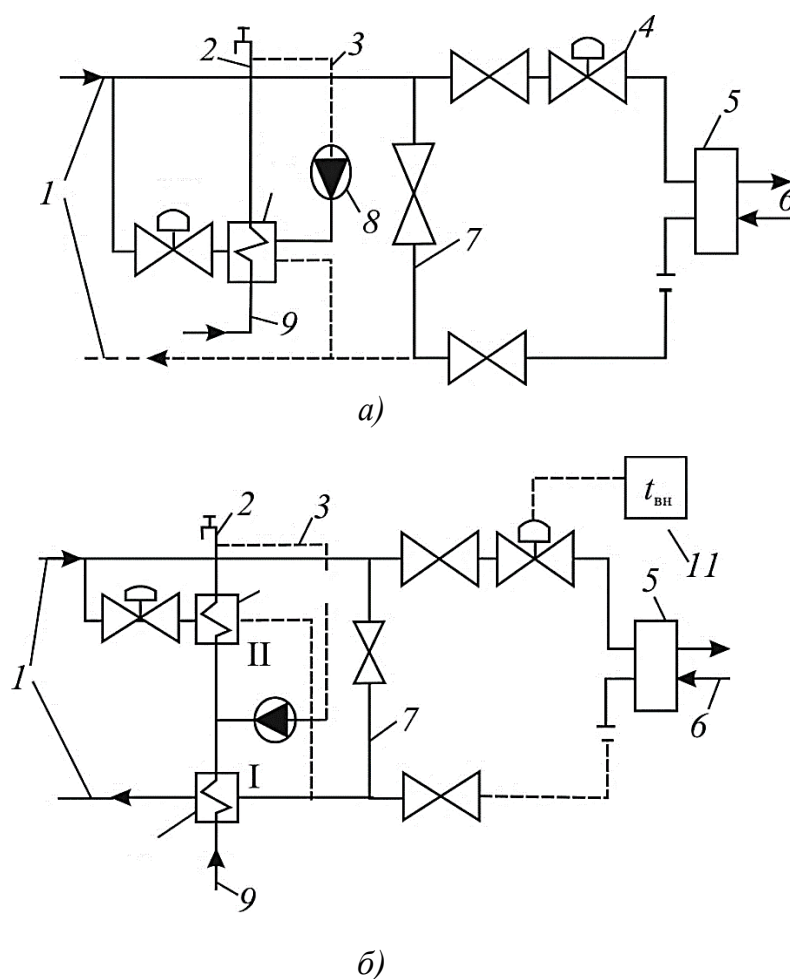
Рис. 4.2. Схемы абонентских вводов с нормальной подачей тепла в систему отопления:
