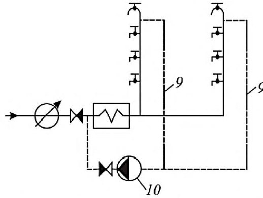
Рис. 3.3. Система с нижней разводкой
