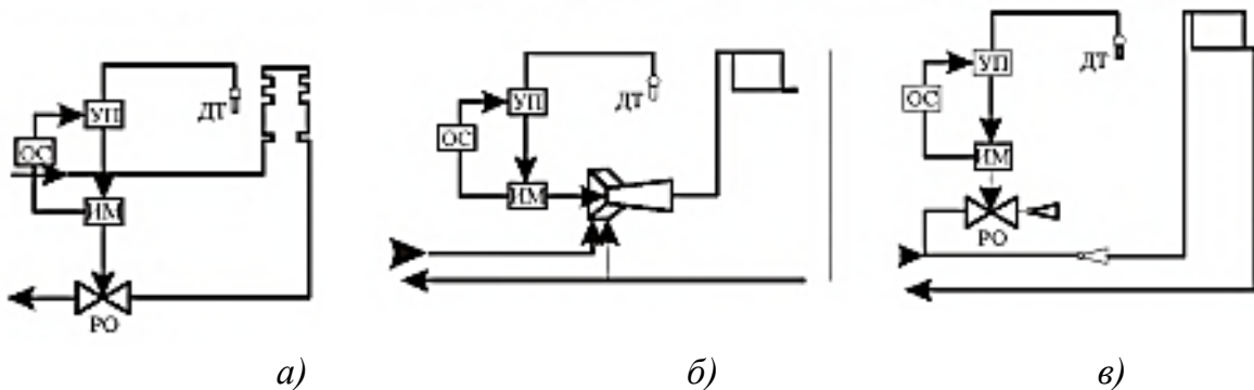
Рис. 5.6. Основные схемы автоматического регулирования отпуска тепла на отопление по внутренней температуре (начало)
