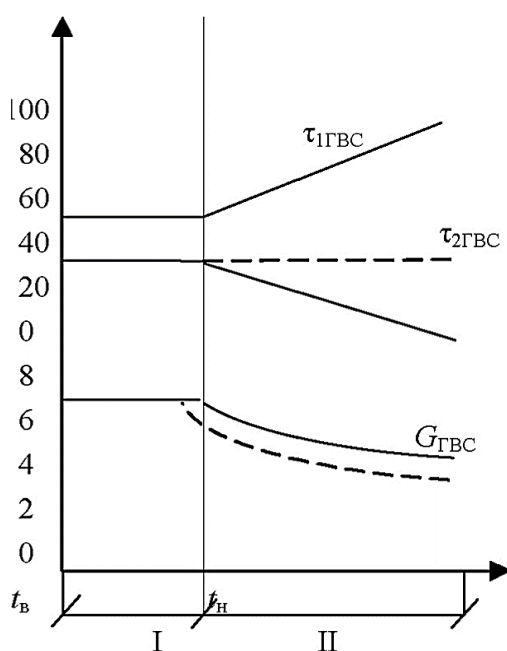
Рис. 4.5. График температур, расходов тепла и сетевой воды на ГВС при параллельной схеме включения подогревателей
