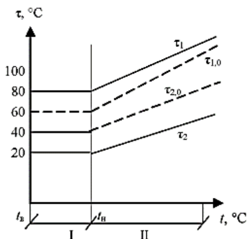
Рис. 4.6 Повышенный температурный график: \tau_{1,0} , \tau_{2,0} – отопительно-бытовой график; \tau_1 , \tau_2 – повышенный график
