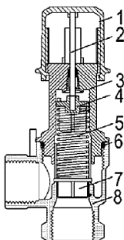
Рис. 7.11. Перепускной клапан
