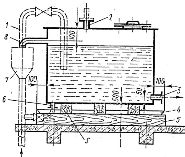
Рис. 3.10. Установка прямоугольного аккумулятора на чердаке:
