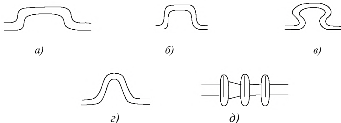
Рис. 7.23. Типы компенсирующих устройств: а – П-образный компенсатор с большой спинкой; б – П-образный компенсатор равносторонний; в – лирообразный компенсатор (бывает гладко загнутый и со складками); г – W-образный компенсатор; д – линзовый компенсатор
