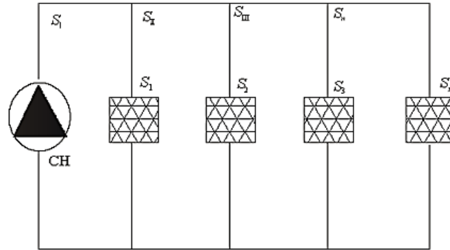
Рис. 6.2 Схема тепловой сети
