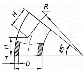
Рис. 7.1. Отвод крутоизогнутый, угол 45^\circ
