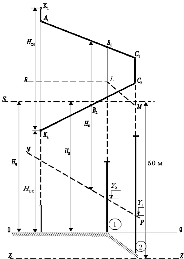
Рис. 8.4. Пример построения пьезометрического графика
