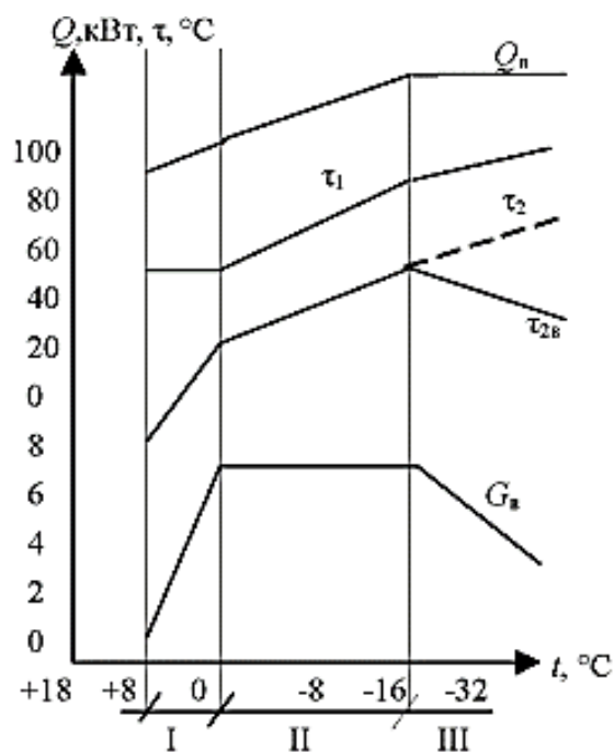
Рис. 4.4 График температур, расходов тепла и сетевой воды при регулировании вентиляционной нагрузки расходом сетевой воды
