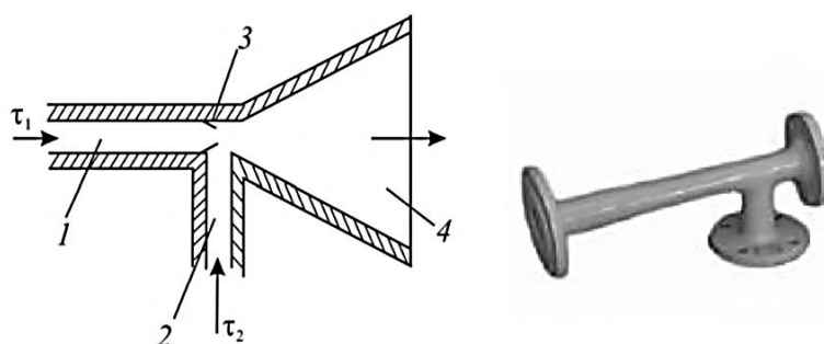
Рис. 2.4. Схема элеватора:
