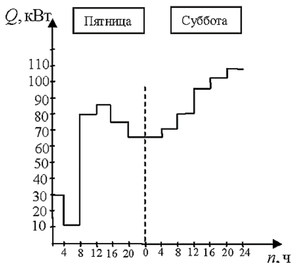
Рис. 2.2. Суточный график расхода тепла на ГВС для жилого района
