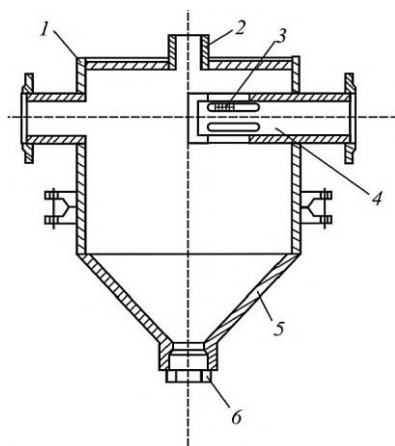
Рис. 5.3. Грязевик
