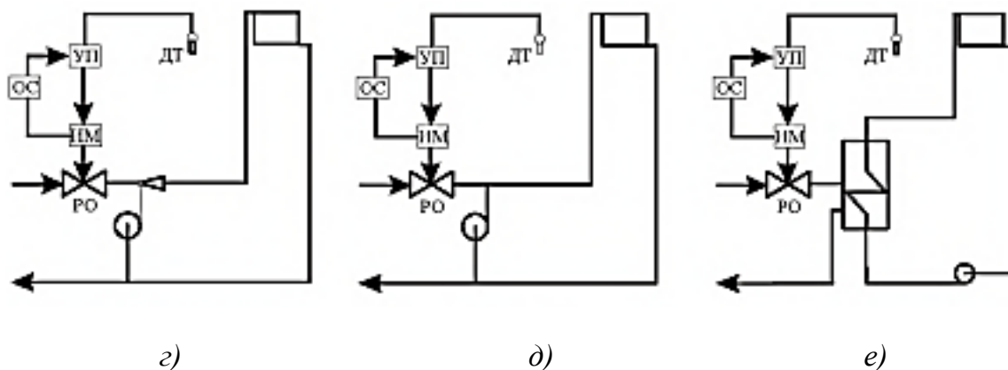
Рис. 5.6. Основные схемы автоматического регулирования отпуска тепла на отопление по внутренней температуре (окончание):
