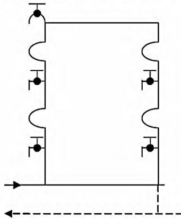
Рис. 3.5. Водоразборный узел с парно закольцованными стояками
