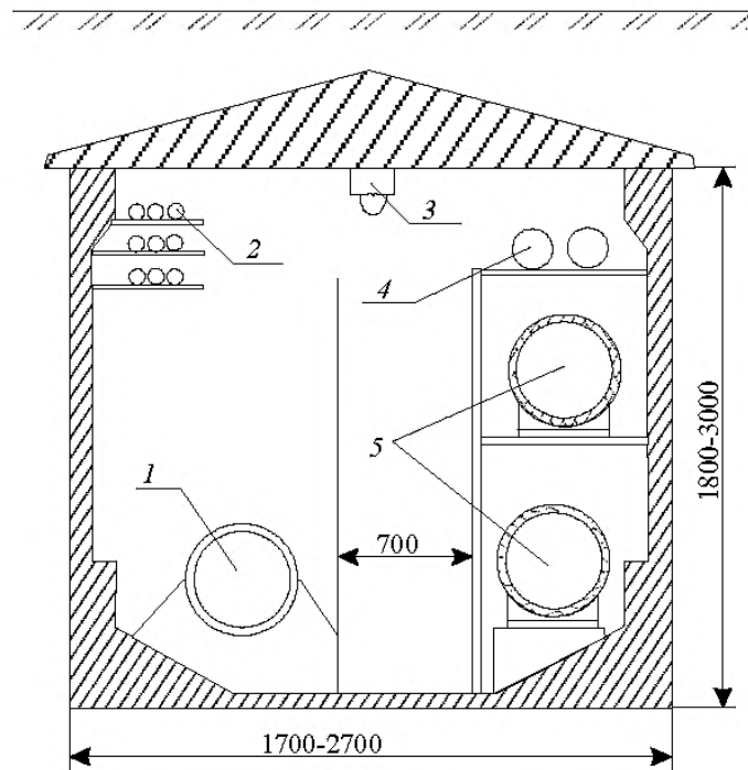
Рис. 8.1. Сечение типового односекционного коллектора: 1 - водопровод; 2 - электрические кабели; 3 - светильник; 4 - ГВС; 5 теплопроводы
