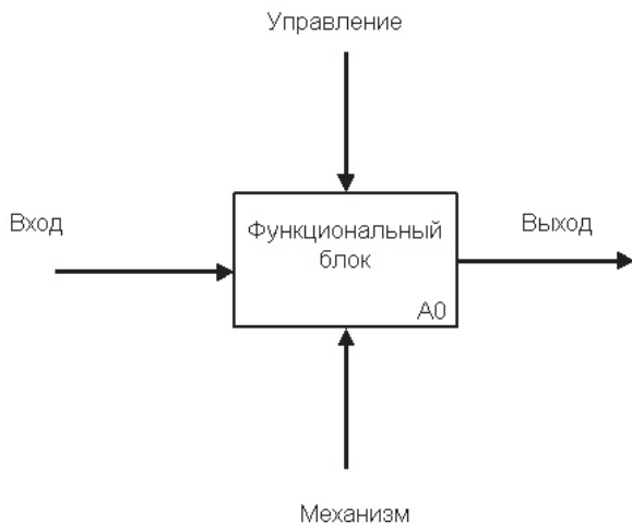
Рис. 4. Типовая IDEF0-диаграмма
