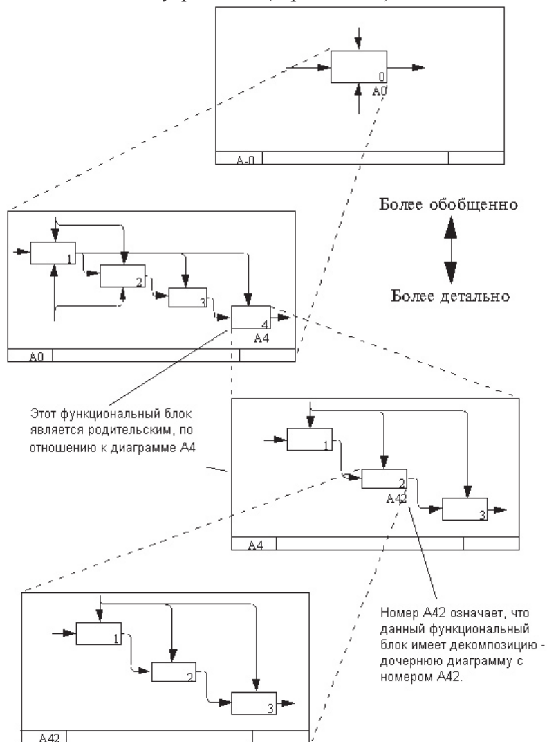
Рис. 5. Иерархическая IDEF0-модель
